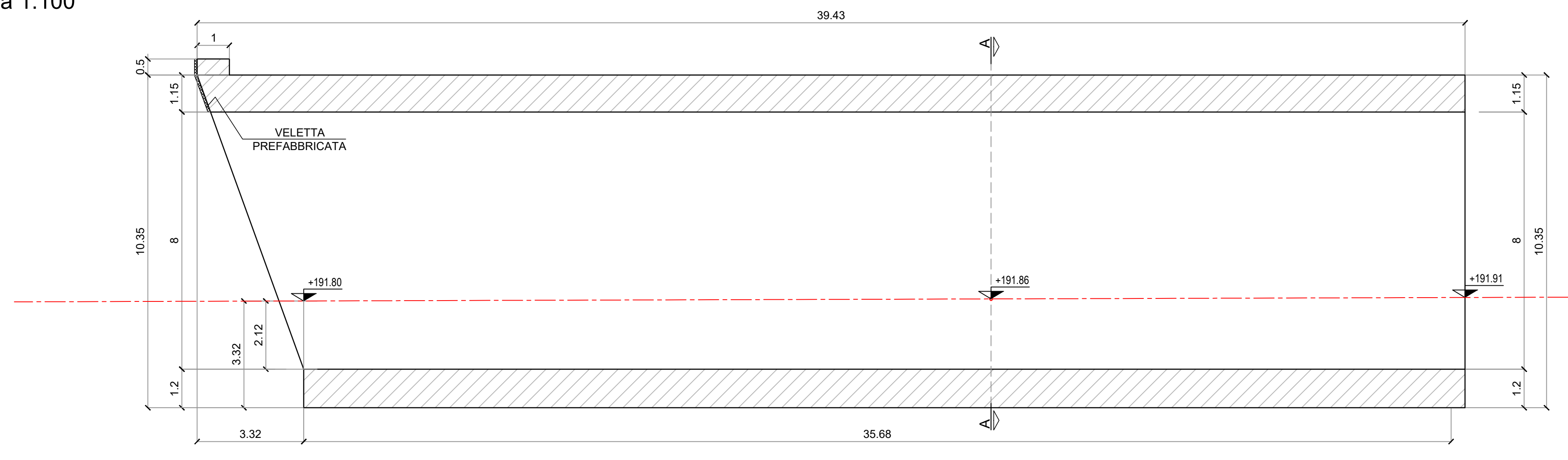
PIANTA SUPERIORE SCATOLARE scala 1:100
