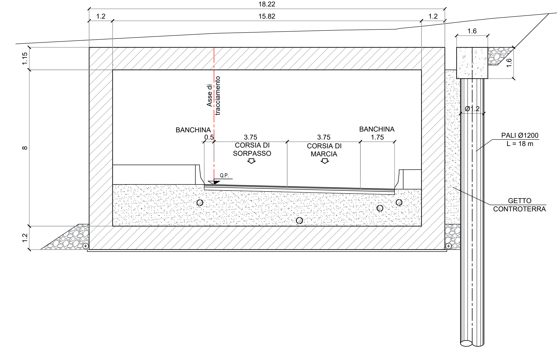
SEZIONE A-A (progr. +4612,92) scala 1:100
