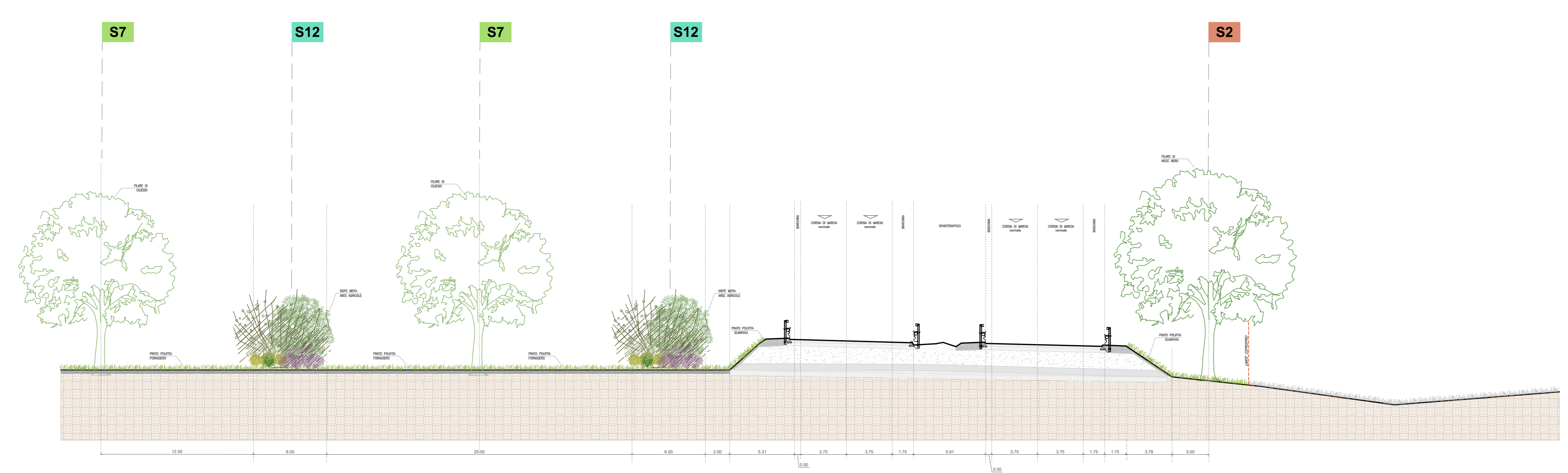
SEZIONE B-B'
