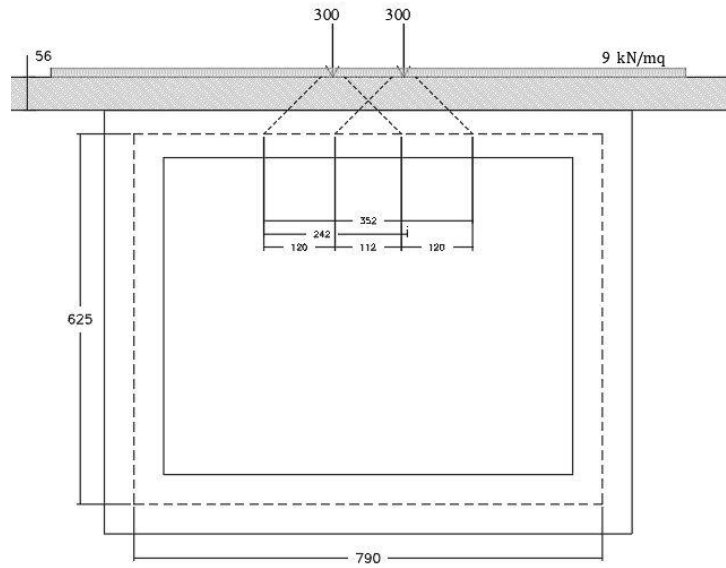
Figura 9.11: Schema delle corsie di marcia su struttura
