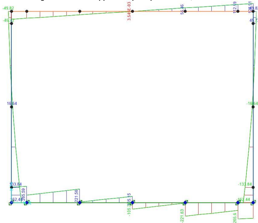
Figura 10.11: Inviluppo SLE quasi permanente, taglio
