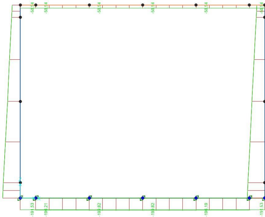
Figura 10.12: Involucro SLE quasi permanente, sforzo normale
