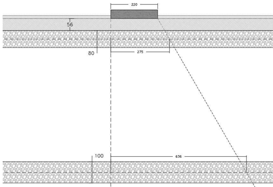
Figura 9.6: Distribuzione del carico veicolare su sezione longitudinale
