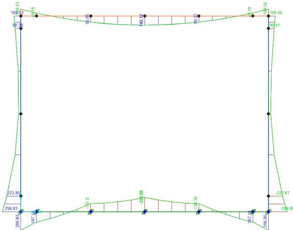
Figura 10.10: Inviluppo SLE quasi permanente, momento
