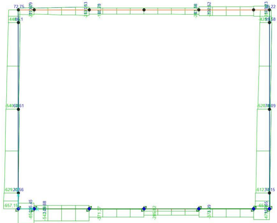
Figura 10.3: Involuppo SLU-SLV, sforzo normale
