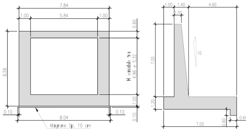
Figura 2-1: Pianta e sezione dell'opera in esame
