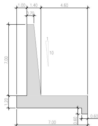
SEZIONE C-C MURO D'ALA - Scala 1:50
