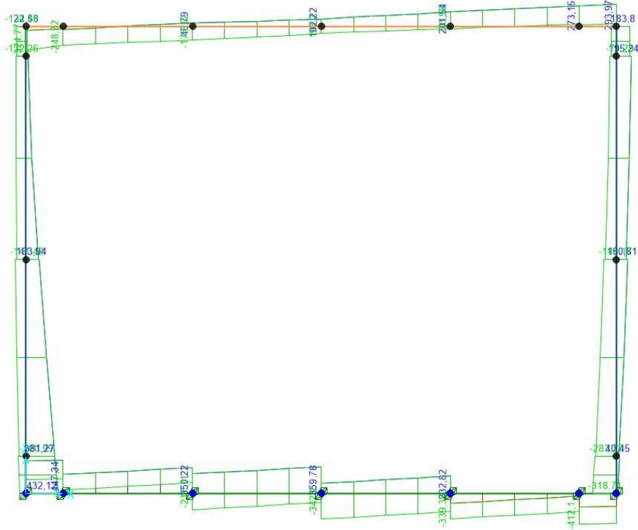
Figura 10.5: Involuppo SLEr-SLD, taglio
