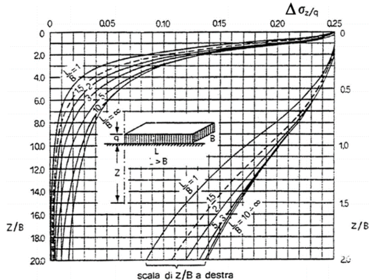
Figura 7-1: Incrementi di tensione \Delta\sigma_z lungo la verticale per lo spigolo di un'area di carico uniforme.
