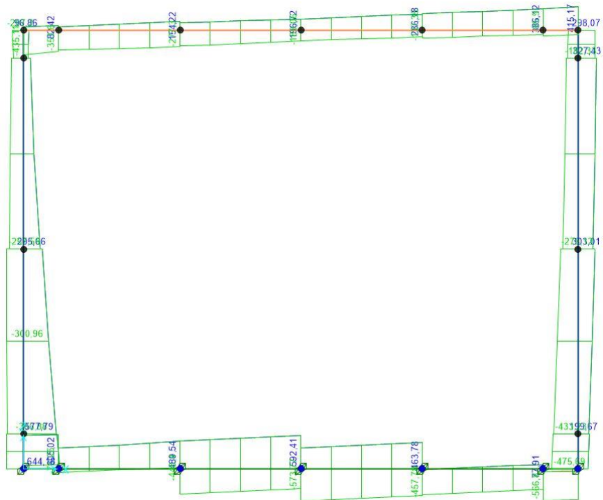
Figura 10.2: Involuppo SLU-SLV, taglio
