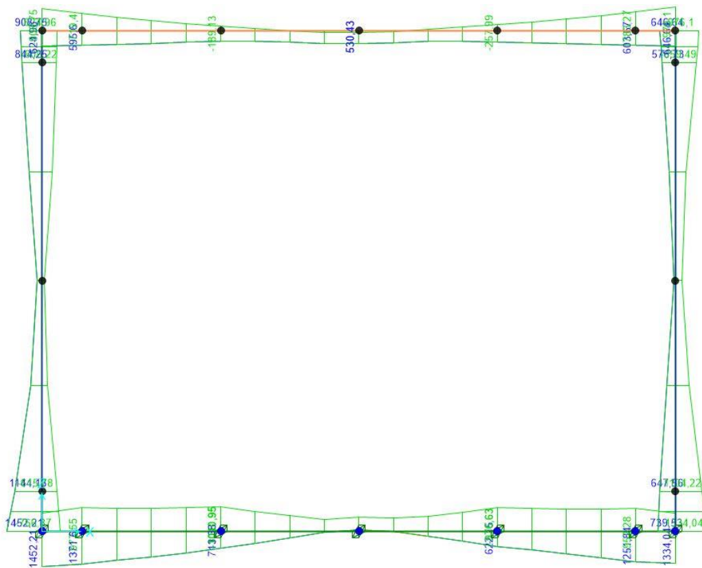
Figura 10.1: Inviluppo SLU-SLV, momento
