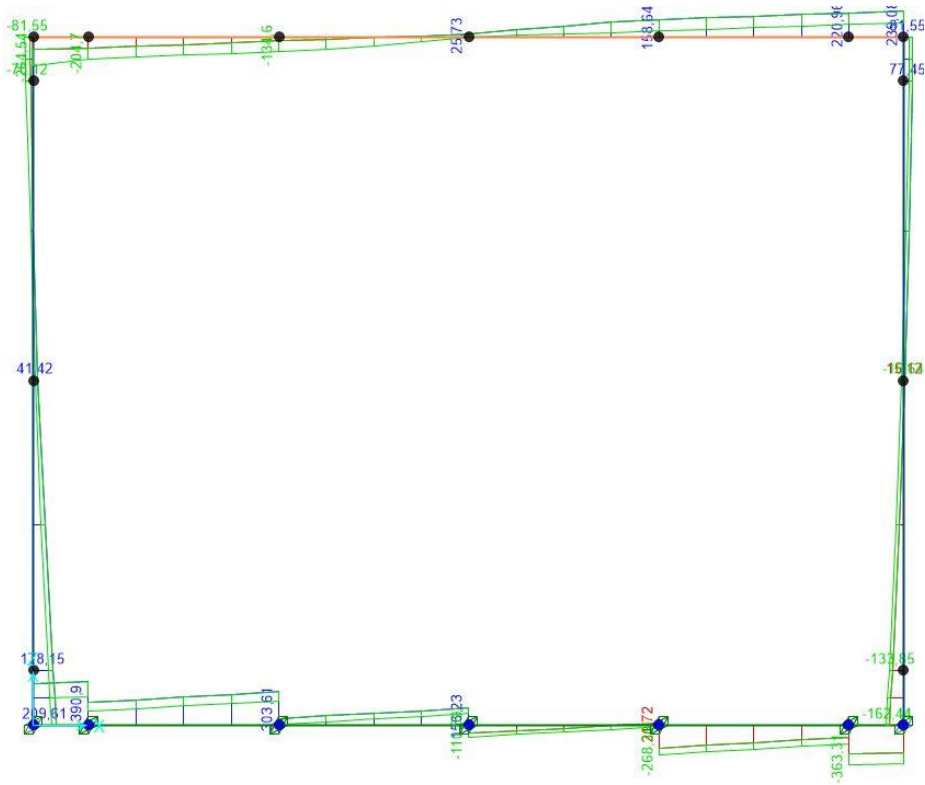
Figura 10.8: Inviluppo SLE frequente, taglio
