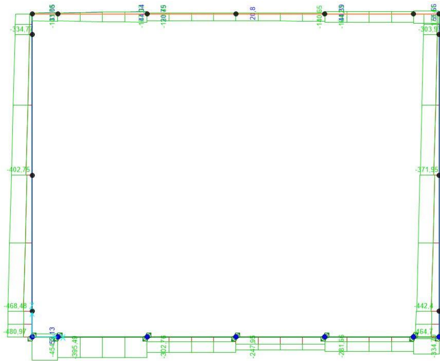
Figura 10.6: Involuppo SLEr-SLD, sforzo normale
