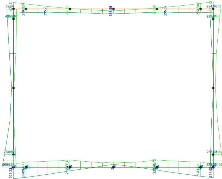
Figura 10.4: Involuppo SLEr-SLD, momento
