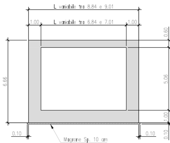
SEZIONE B-B SOTTOPASSO - Scala 1:50
