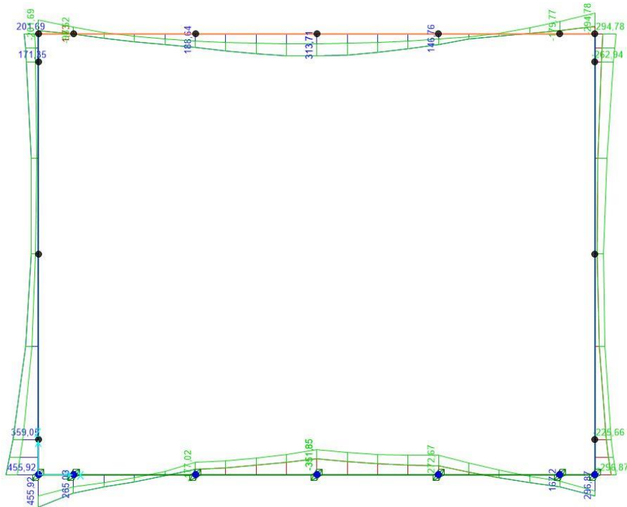
Figura 10.7: Involuppo SLE frequente, momento
