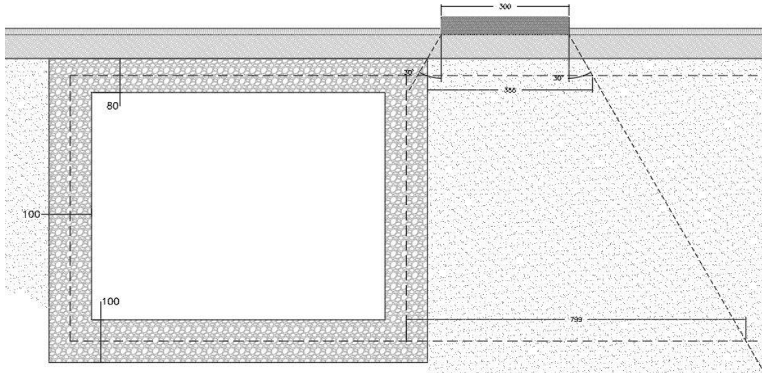
Figura 9.5: Distribuzione del carico veicolare su sezione trasversale
