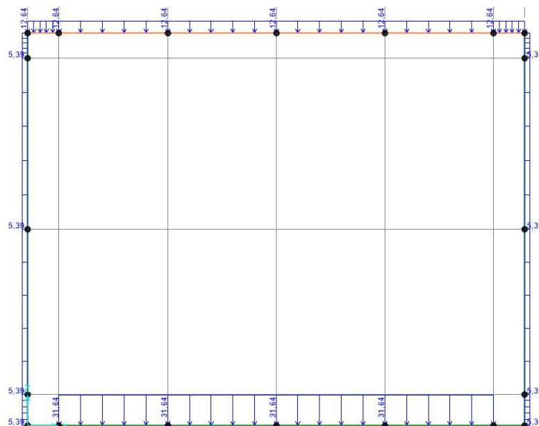
Figura 9.2: Peso di pavimentazione stradale
