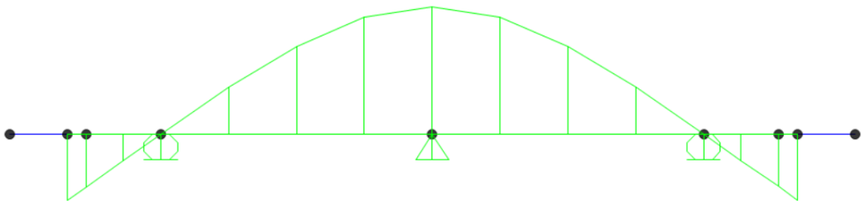
LDI della reazione sull'appoggio centrale
