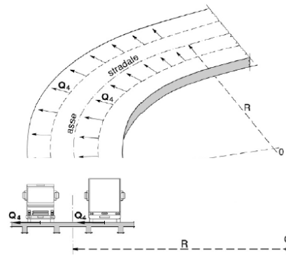
Azione centrifuga per impalcati a 3 e 2 colonne
