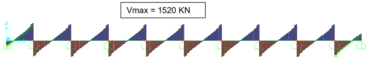
Sollecitazioni SLU
