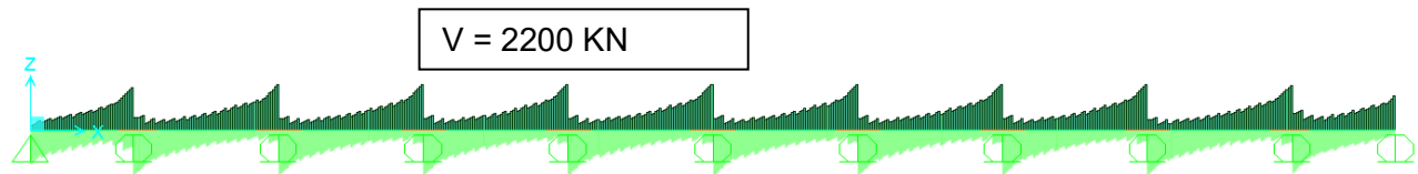
Sollecitazioni SLU
