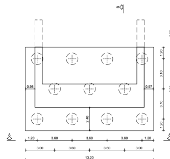
Figura 1.5 Pianta palificata Spalla B
