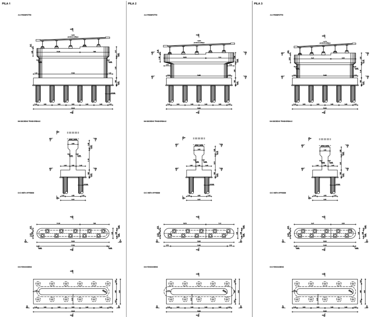
Figura 1.6 Pile
