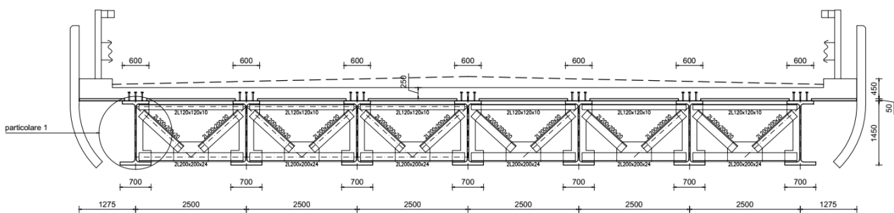
Sezione tipologica
