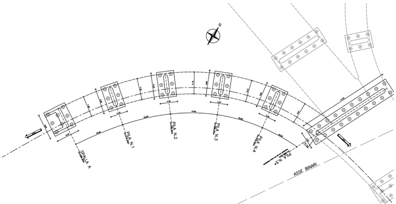
Figura 1.4 Fondazioni del viadotto
