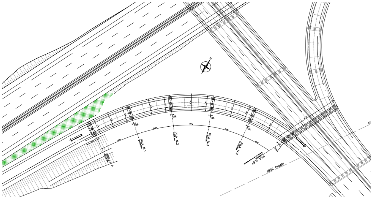
Figura 1.2 Planimetria del viadotto
