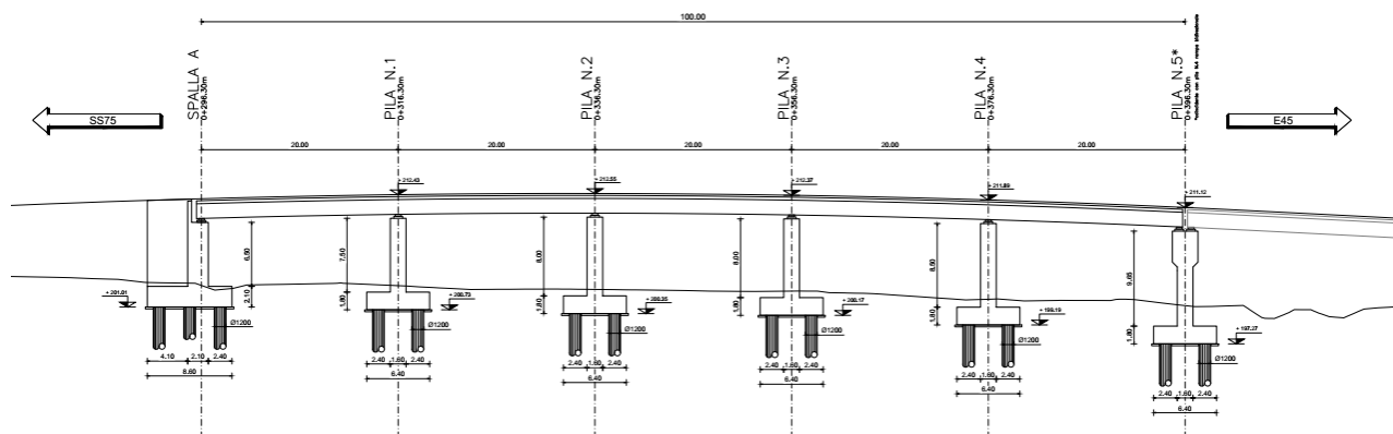
Figura 3.1 Profilo del viadotto
