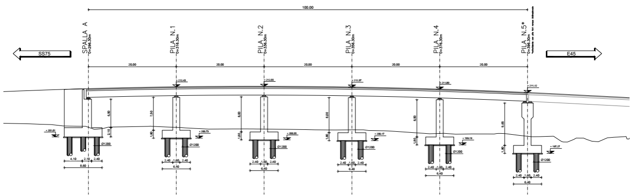
Figura 1.3 Profilo del viadotto
