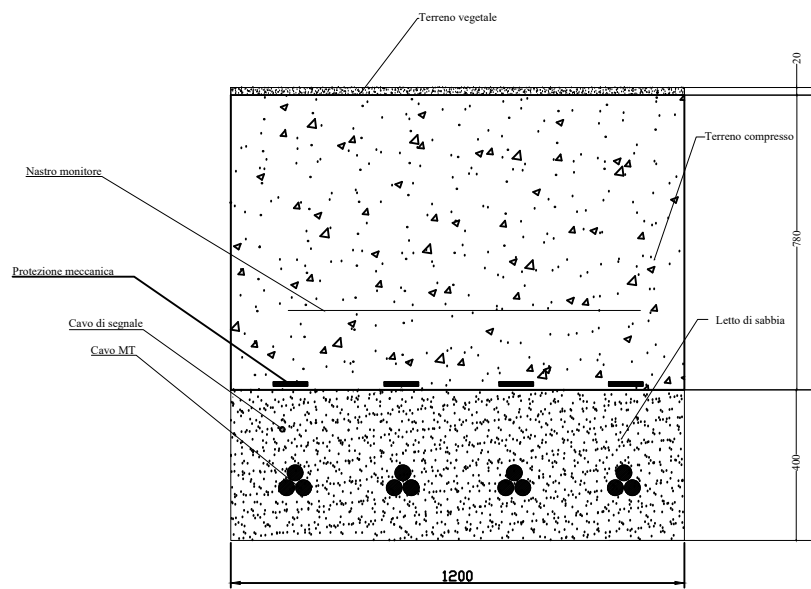
Particolare cavidotto MT su terreno
