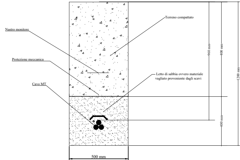
Particolare cavidotto MT su pista
