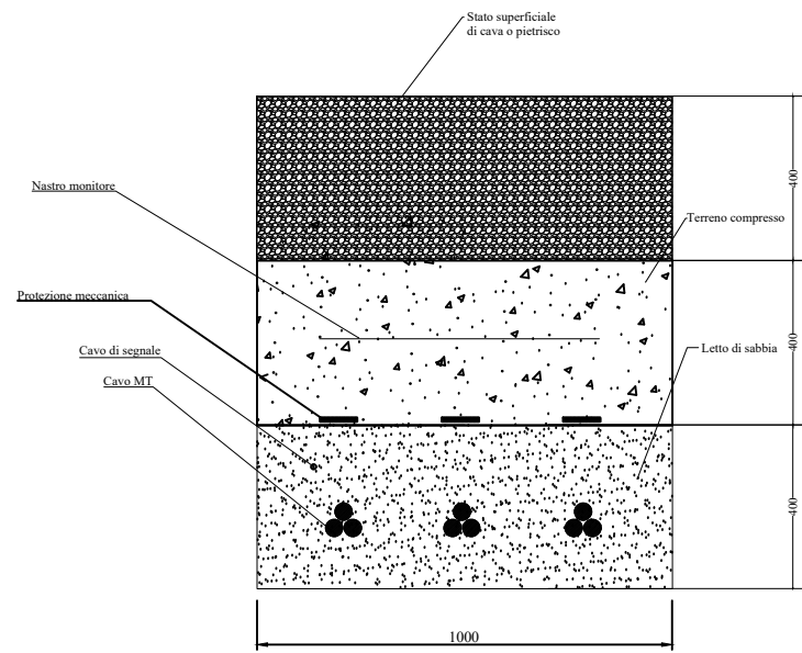
Particolare cavidotto MT su pista
