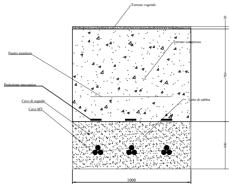
Particolare cavidotto MT su terreno
