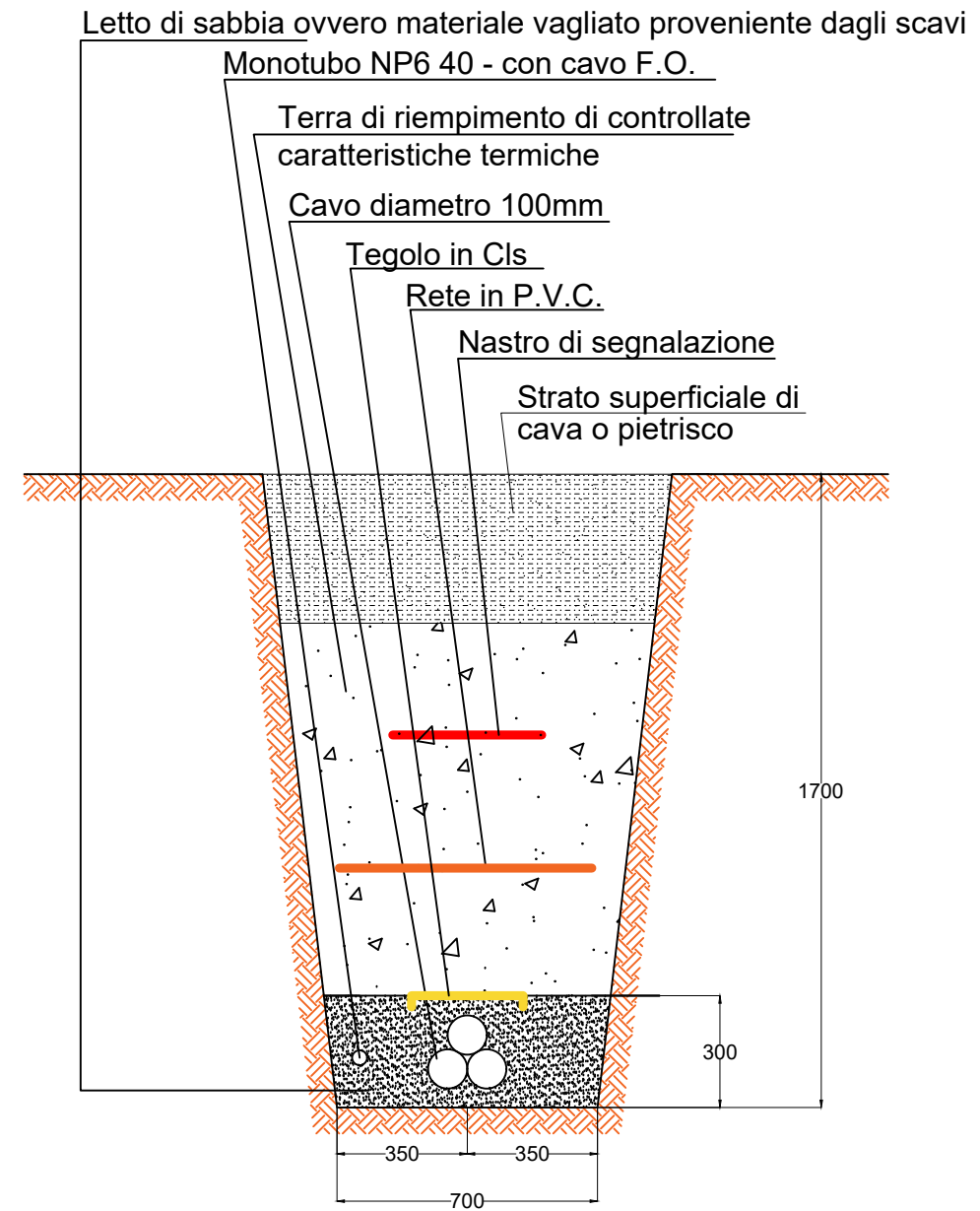
Particolare cavidotto AT su pista
