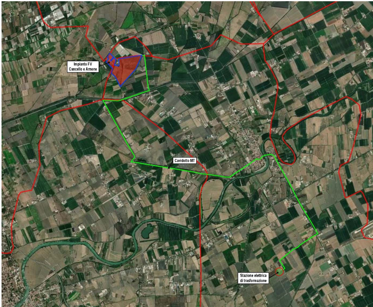
Figura 4. Ortofoto con identificazione dell'area di impianto e del tracciato del cavidotto
