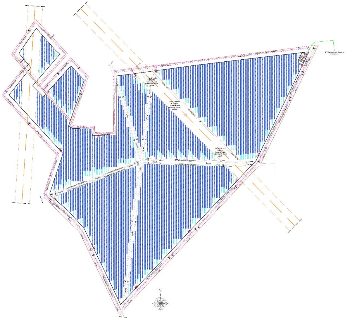
Figura 2. Planimetria generale di Impianto
