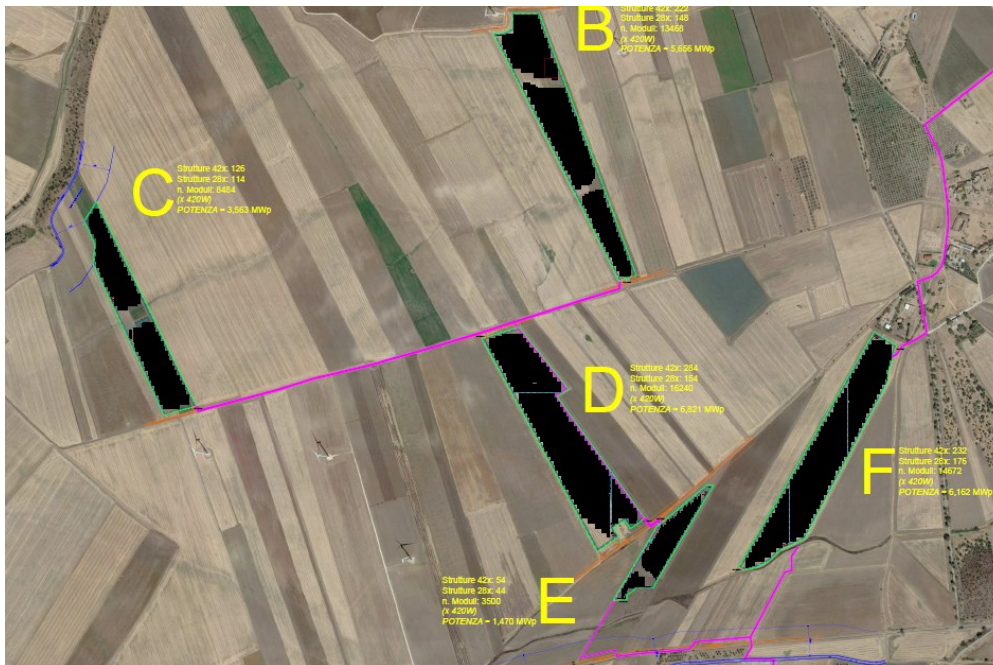
Figura 4 – Layout di impianto dell’Area B-C-D-E e F
