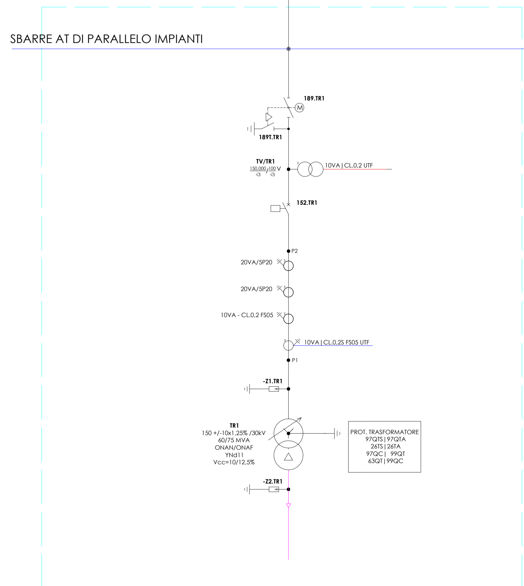
Impianto Green Genius Italy Utility5 - Zezza 2 Potenza 60 MW 201900770
