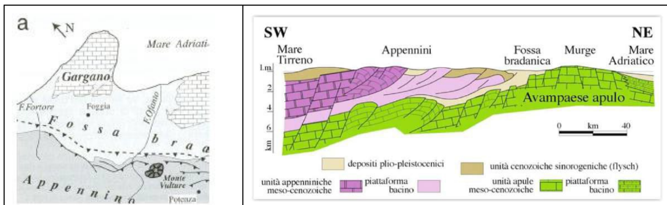
In figura: Schema tettonico e stratigrafico - liberamente tratto da Guide Geologiche Regionali n-9
