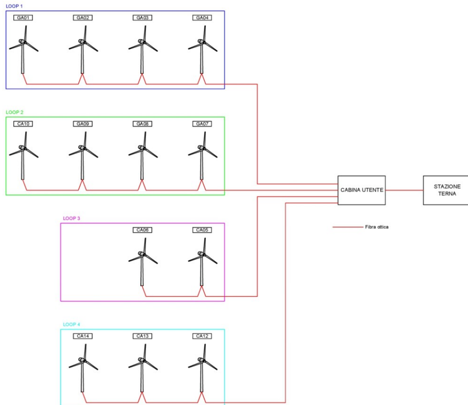
Figura 3 - Schema fibra ottica
