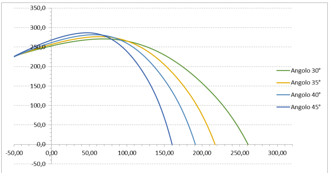
Grafico della traiettoria di un frammento di pala lungo 10 mt
