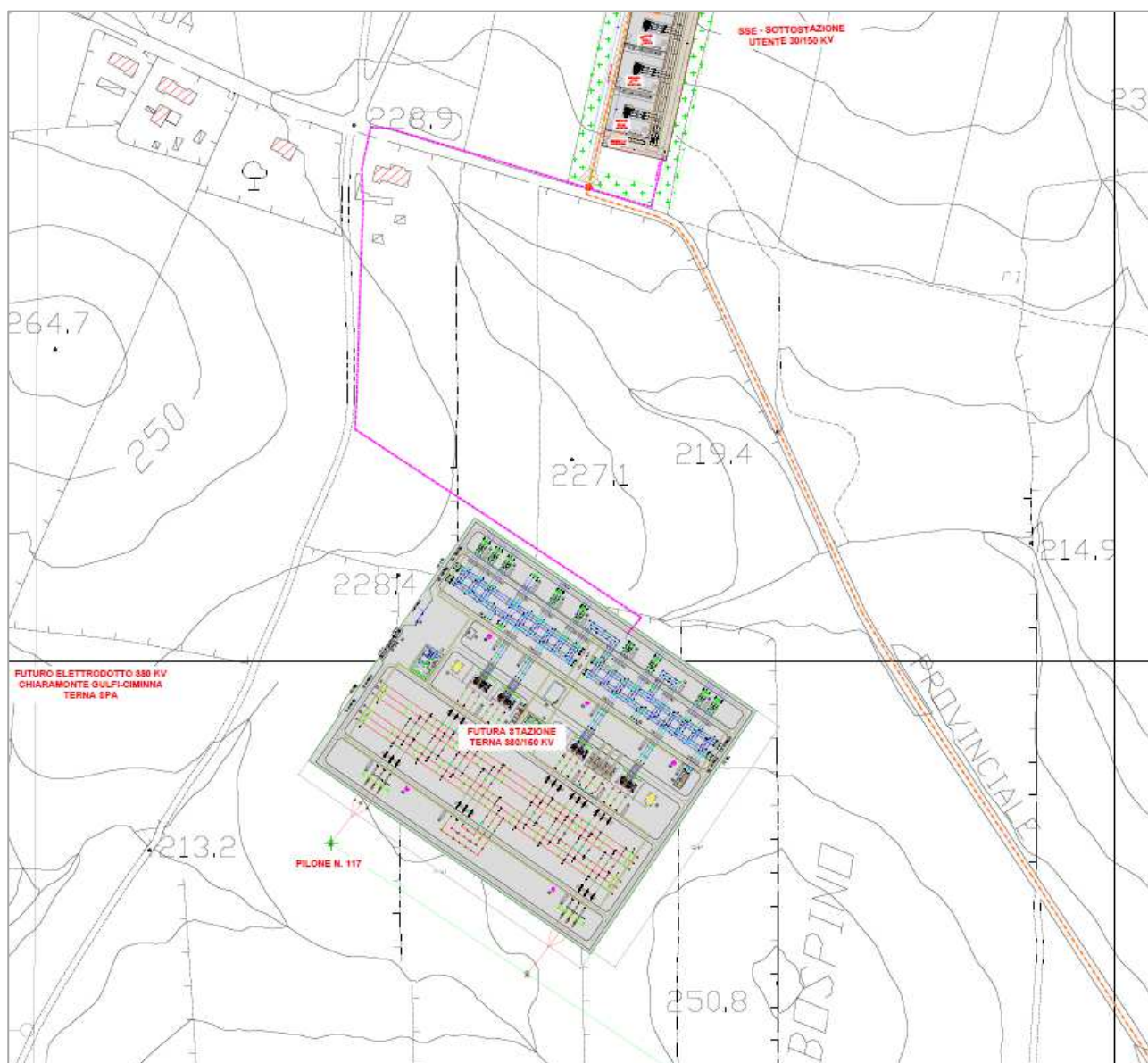
Tracciato elettrodotto AT interrato su planimetria catastale
