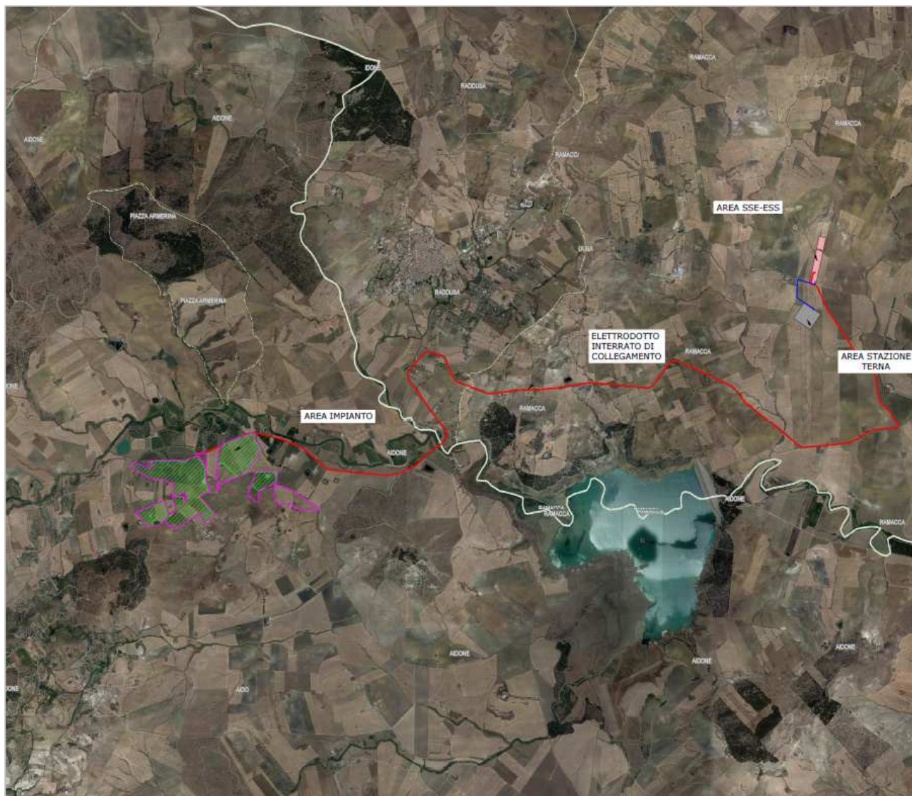
Inquadramento aree e opere lineari su ortofoto (Elaborato FR-AIDONE-AFV-PD-D-1.4.0.0)
