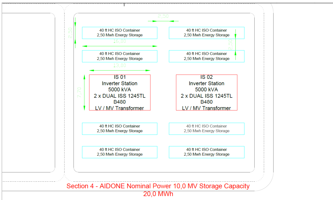
Lay-out ESS
