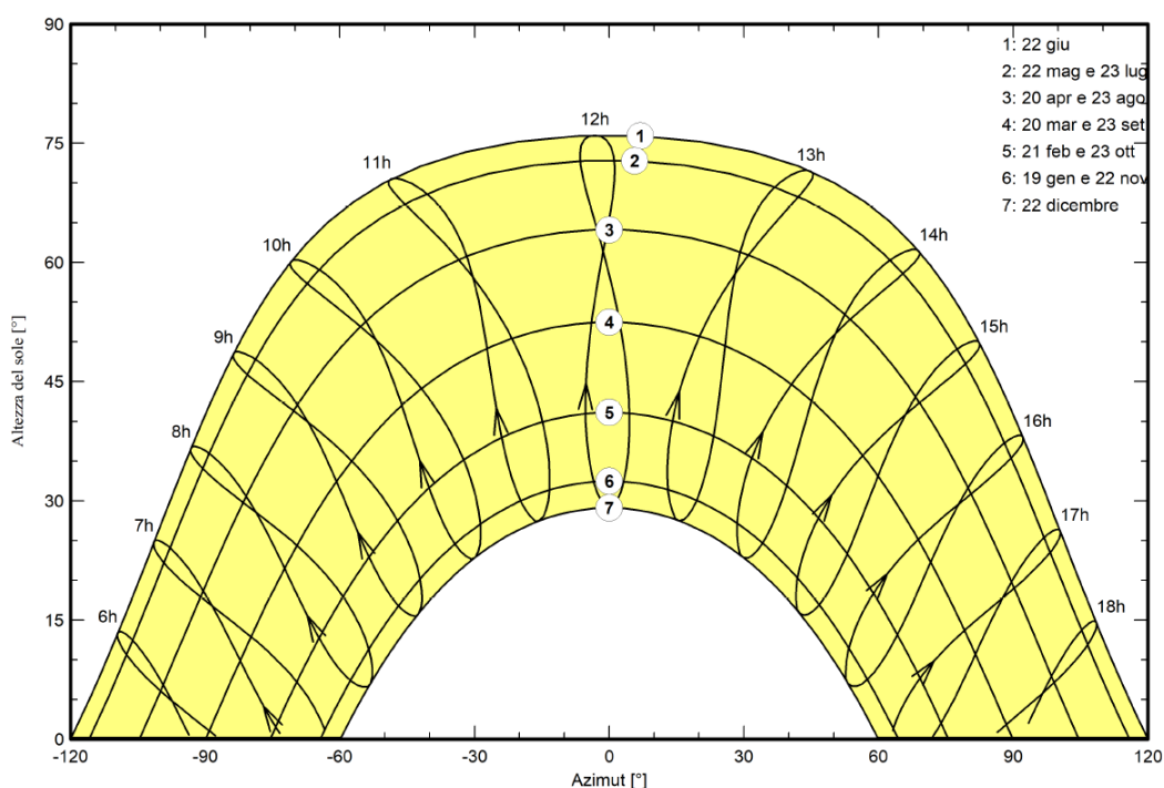
Diagramma clinometrico
