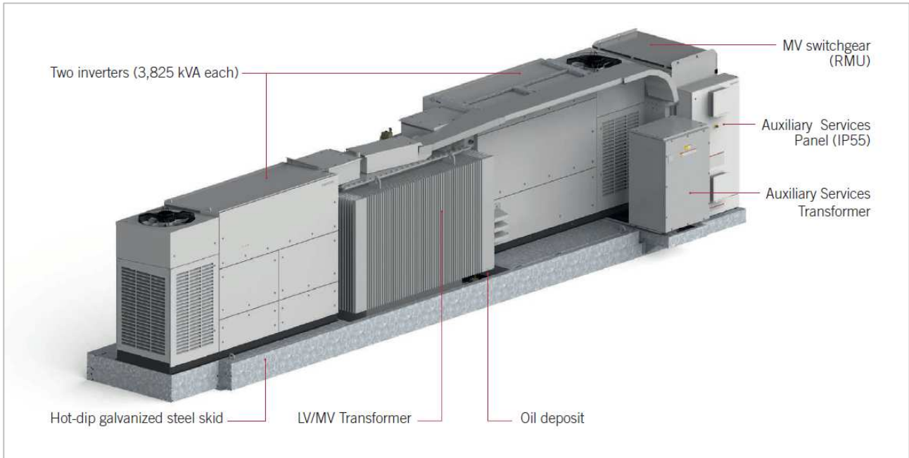
Esempio di Power Station Sun FSK C Series 7650 nella configurazione 2 inverter + 1 trasformatore MT/BT
