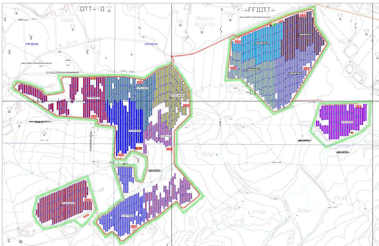
PLANIMETRIA IMPIANTO CON SUDDIVISIONE IN CAMPI - FR-AIDONE-AFV-PD-D-3.2.2.0
