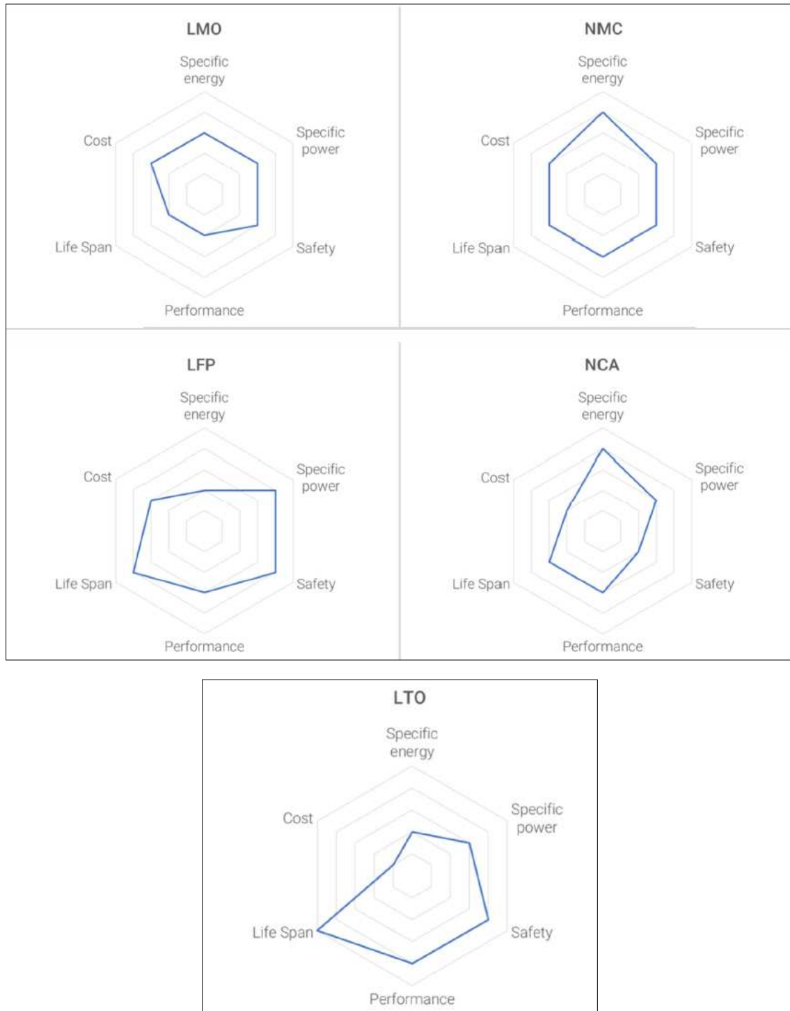
Caratteristiche delle tecnologie litio
