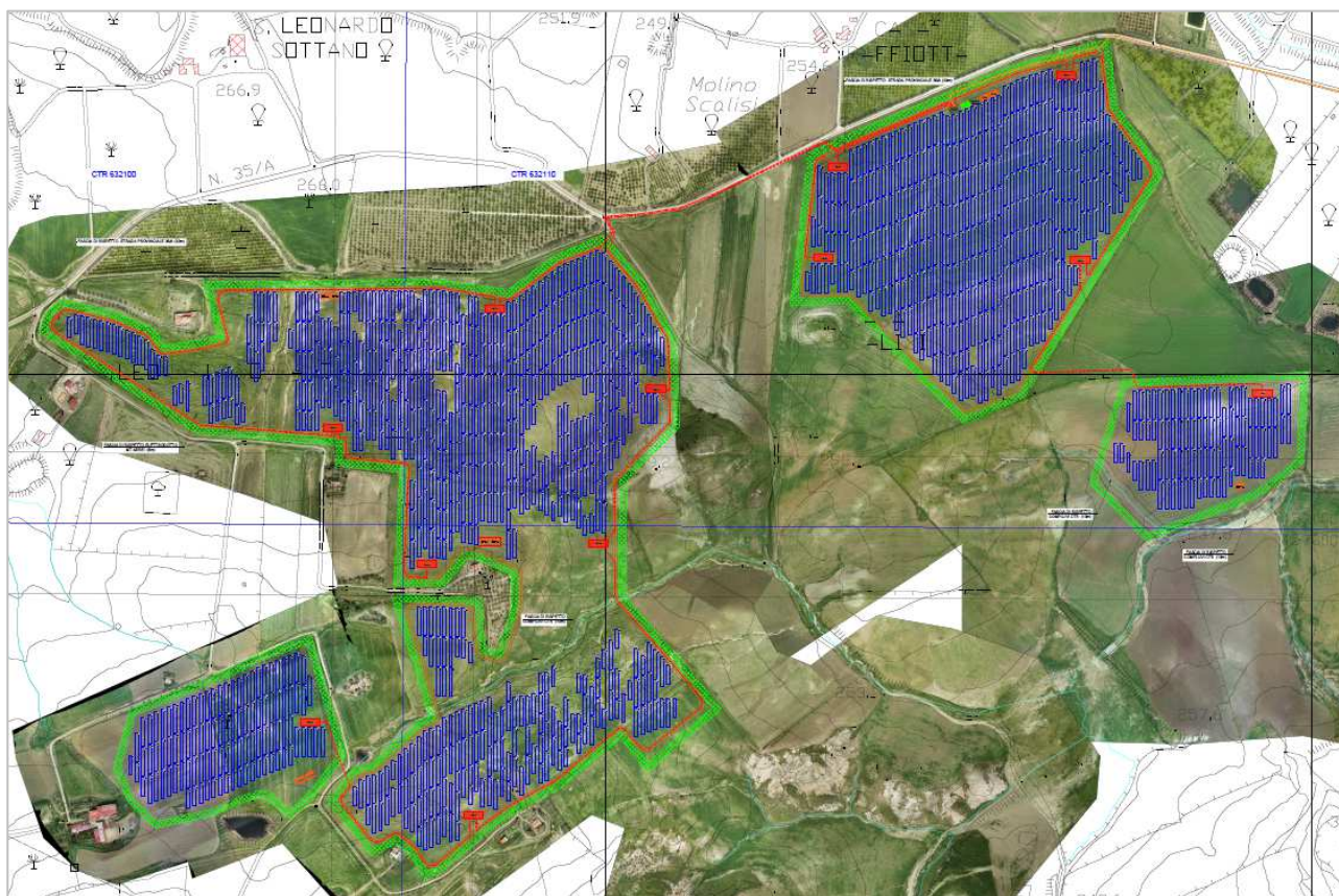
PLANIMETRIA GENERALE DI IMPIANTO SU ORTOFOTO FR-AIDONE-AFV-PD-D-3.2.1.2
