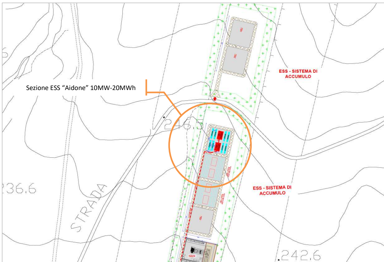
Lay-out Sistema di Accumulo (ESS) – Sezione 2 "Aidone"
