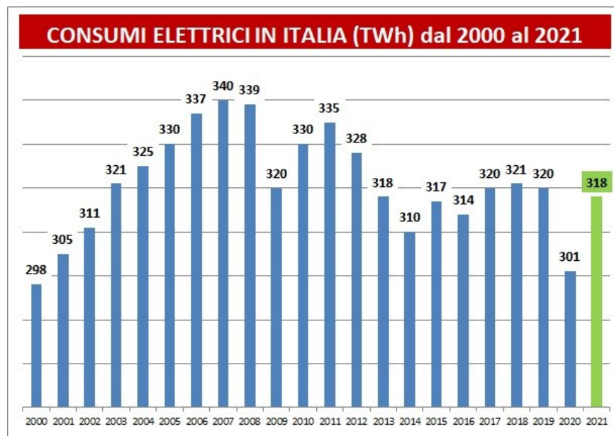
Figura 1 – Consumi elettrici nazionali
