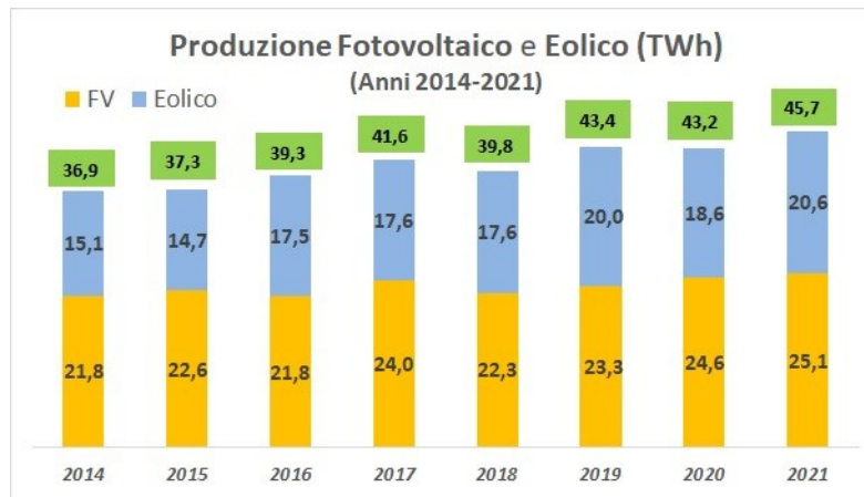
Figura 5 – Produzione Fotovoltaico ed eolico
