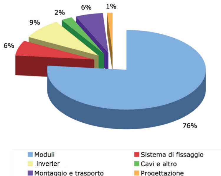
Figura 13 - Ripartizione dei costi di investimento per un impianto fotovoltaico di grandi dimensioni.
