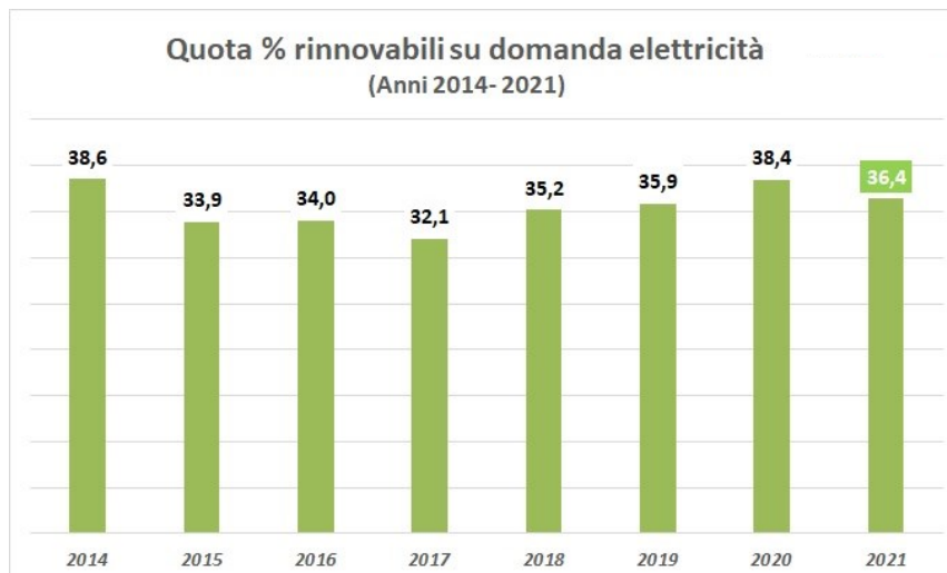
Figura 3 – Percentuale quota rinnovabili su domanda elettricità
