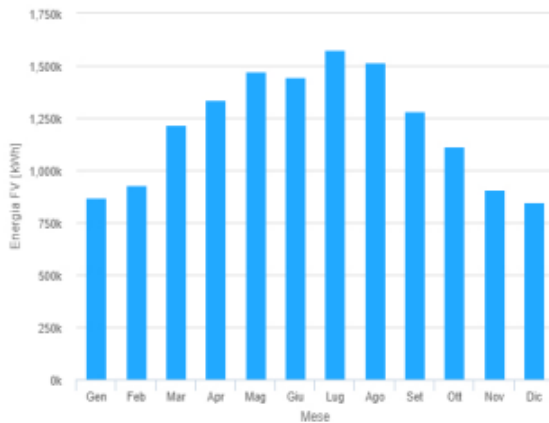
Figura 10 - Energia e Irraggiamento mensile nel piano fisso
