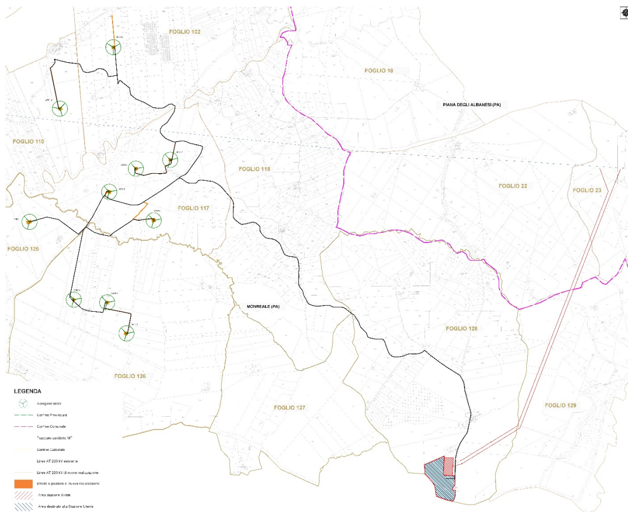
Figura 4 – Layout su Catastale dell'area d'impianto
