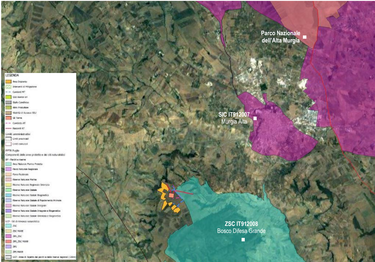
Figura 13-8: Componenti aree protette e siti naturalistici - individuazione di BP e UCP nell'area di impianto
