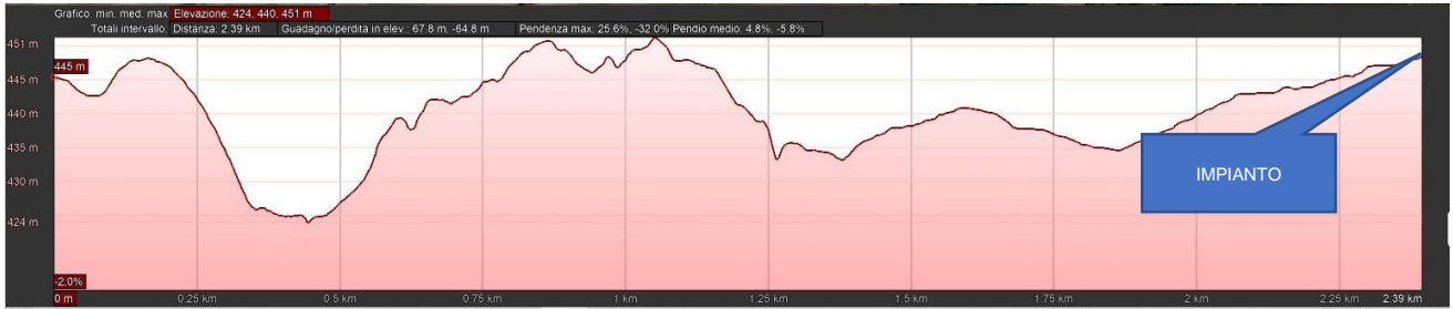
Figura 15-12: Profilo altimetrico dal punto di vista 02 verso l'impianto
