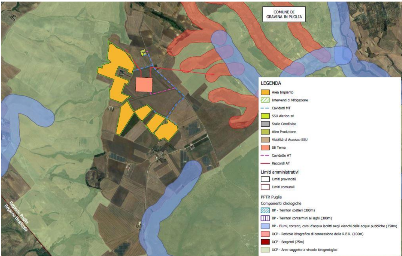
Figura 13-6: Componenti Idrologiche - individuazione di BP e UCP nell'area di impianto
