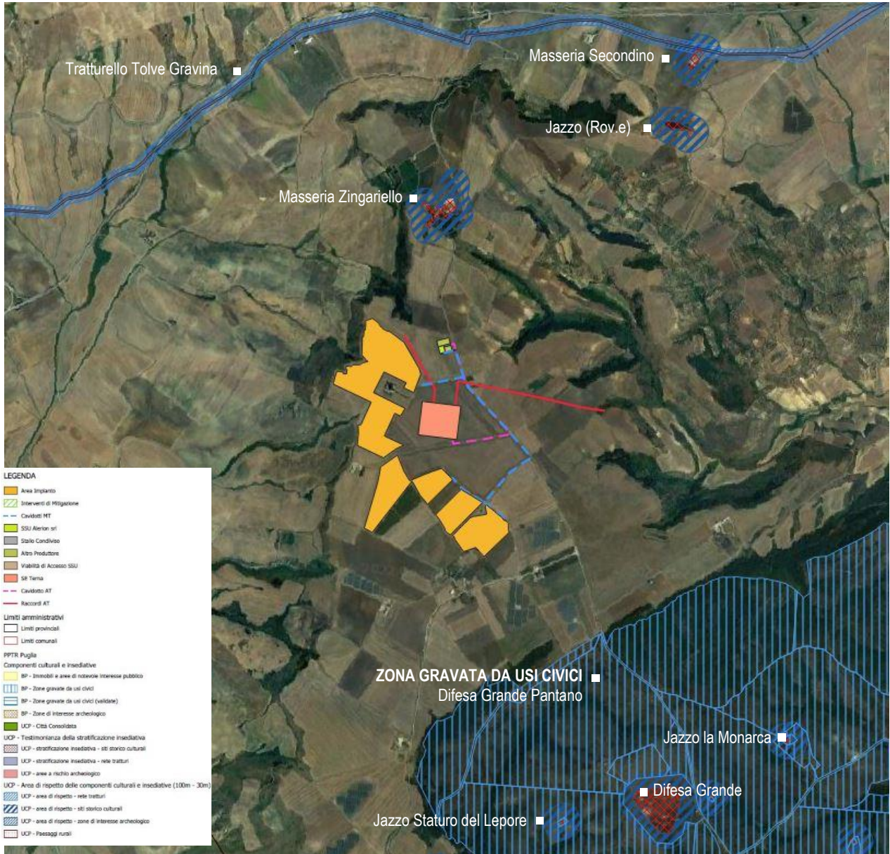
Figura 13-10: Componenti Culturali e Insediative - individuazione di BP e UCP nelle immediate vicinanze dell'area di impianto
