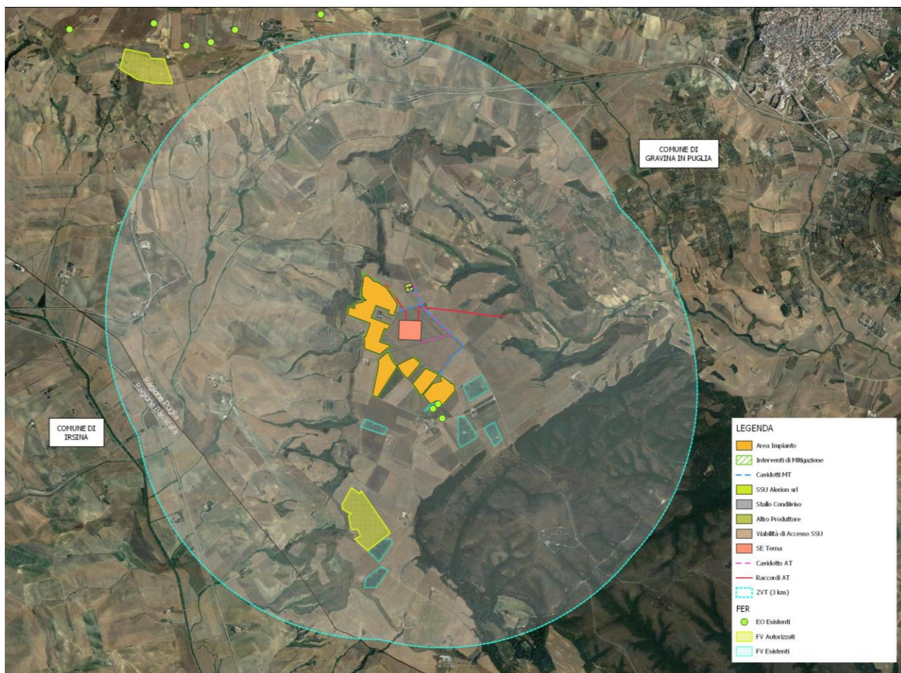
Figura 16-3: Zona di Visibilità Teorica 3 Km con impianti FER esistenti ed autorizzati
