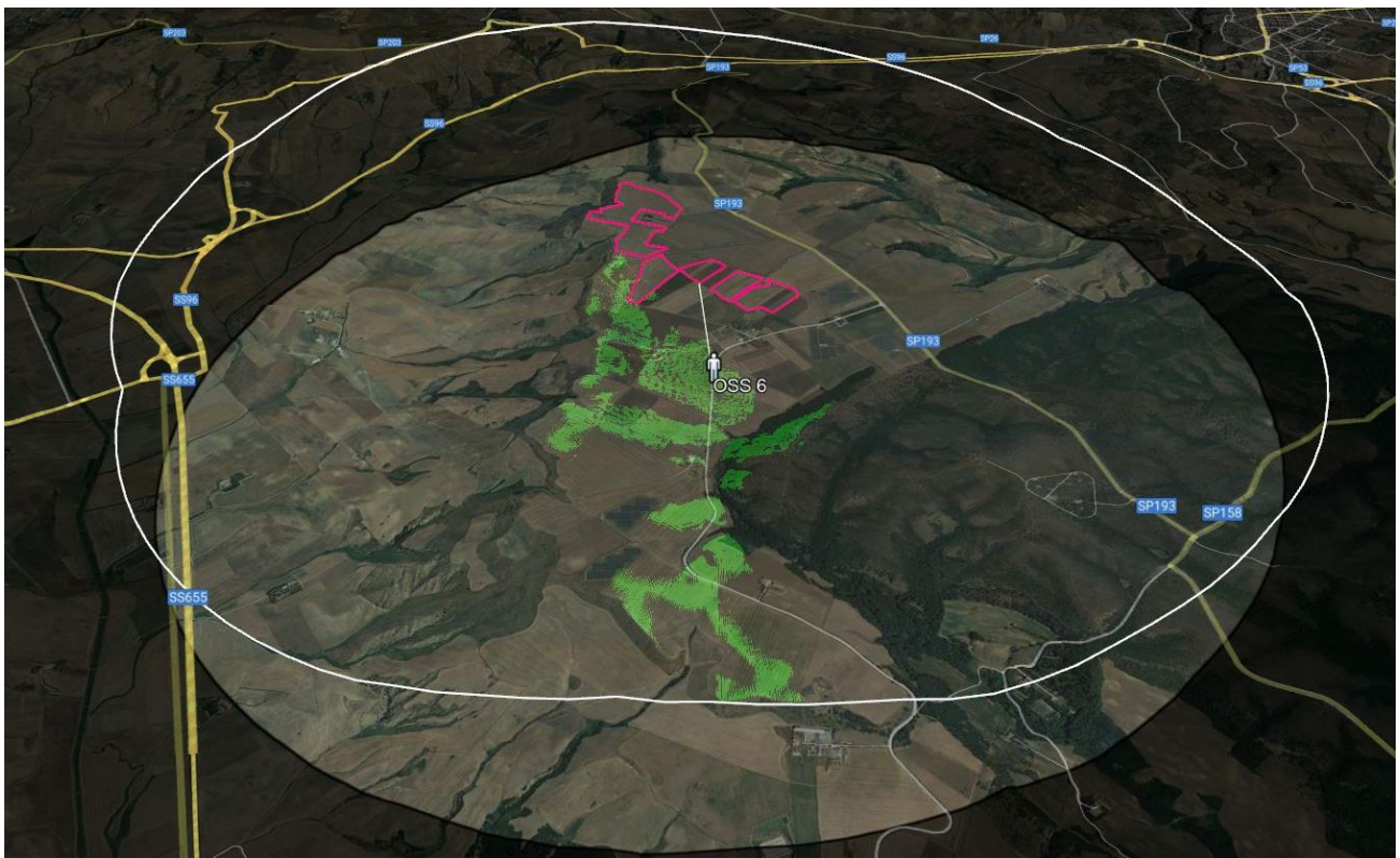
Figura 16-20: OSSERVATORE 6: Area di visibilità teorica
