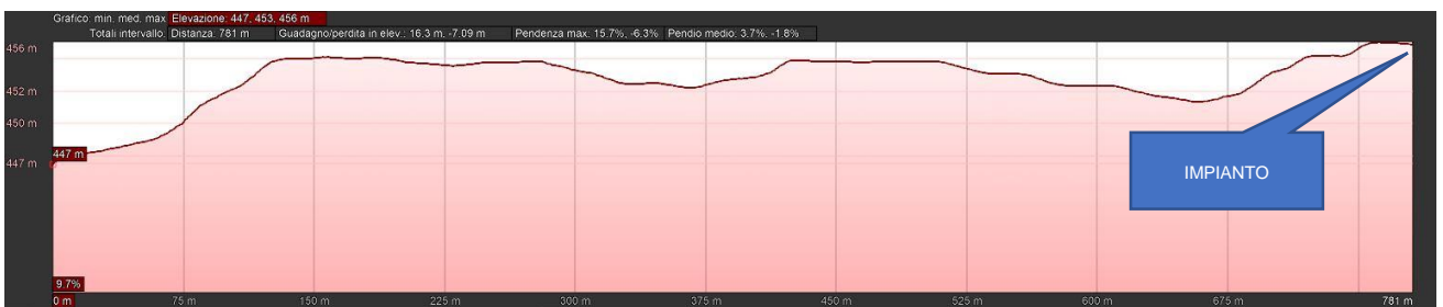
Figura 15-15: Profilo altimetrico dal punto di vista 05 verso l'impianto
