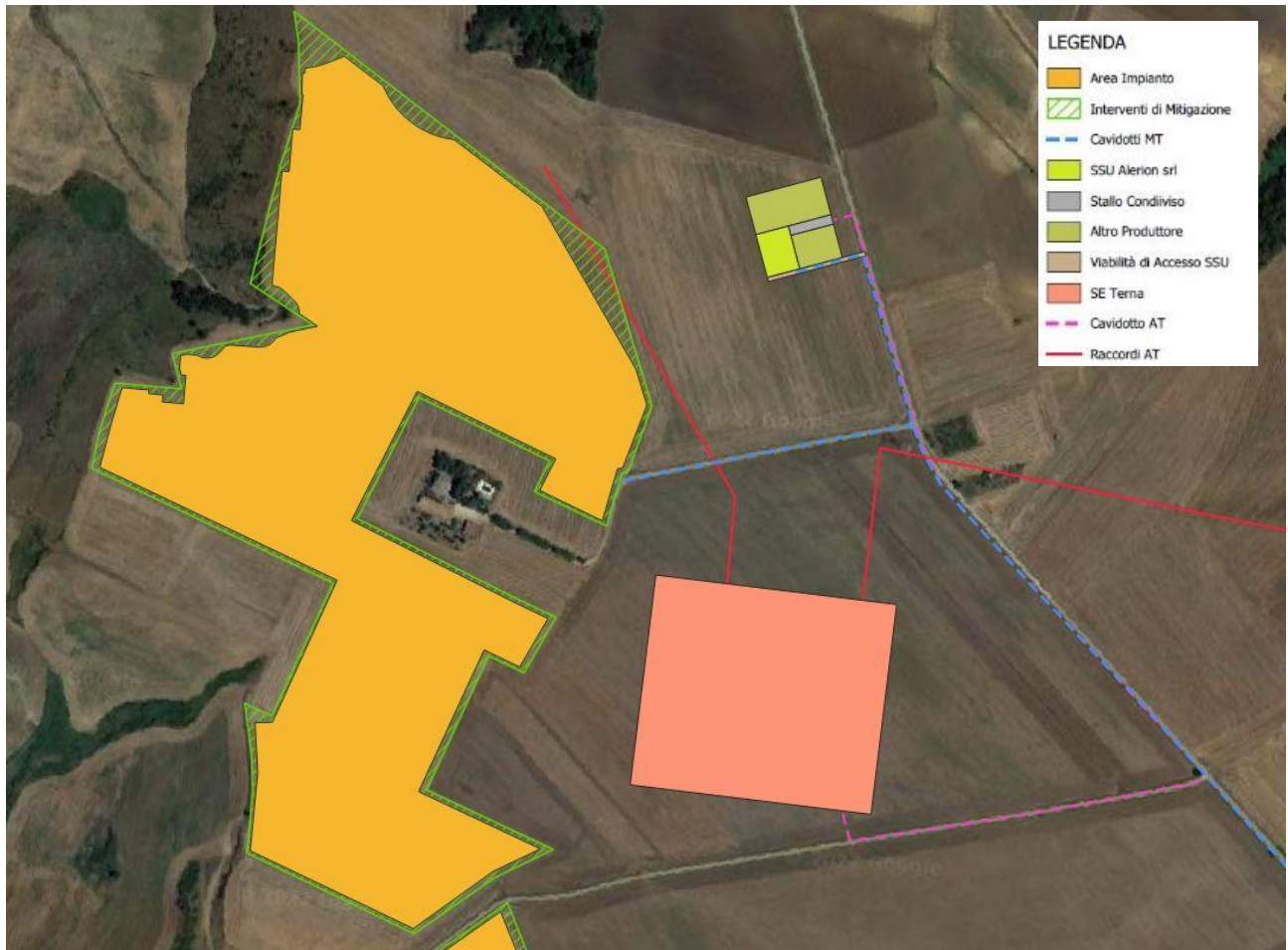
Figura 9-3: Inquadramento delle opere di connessione su ortofoto
