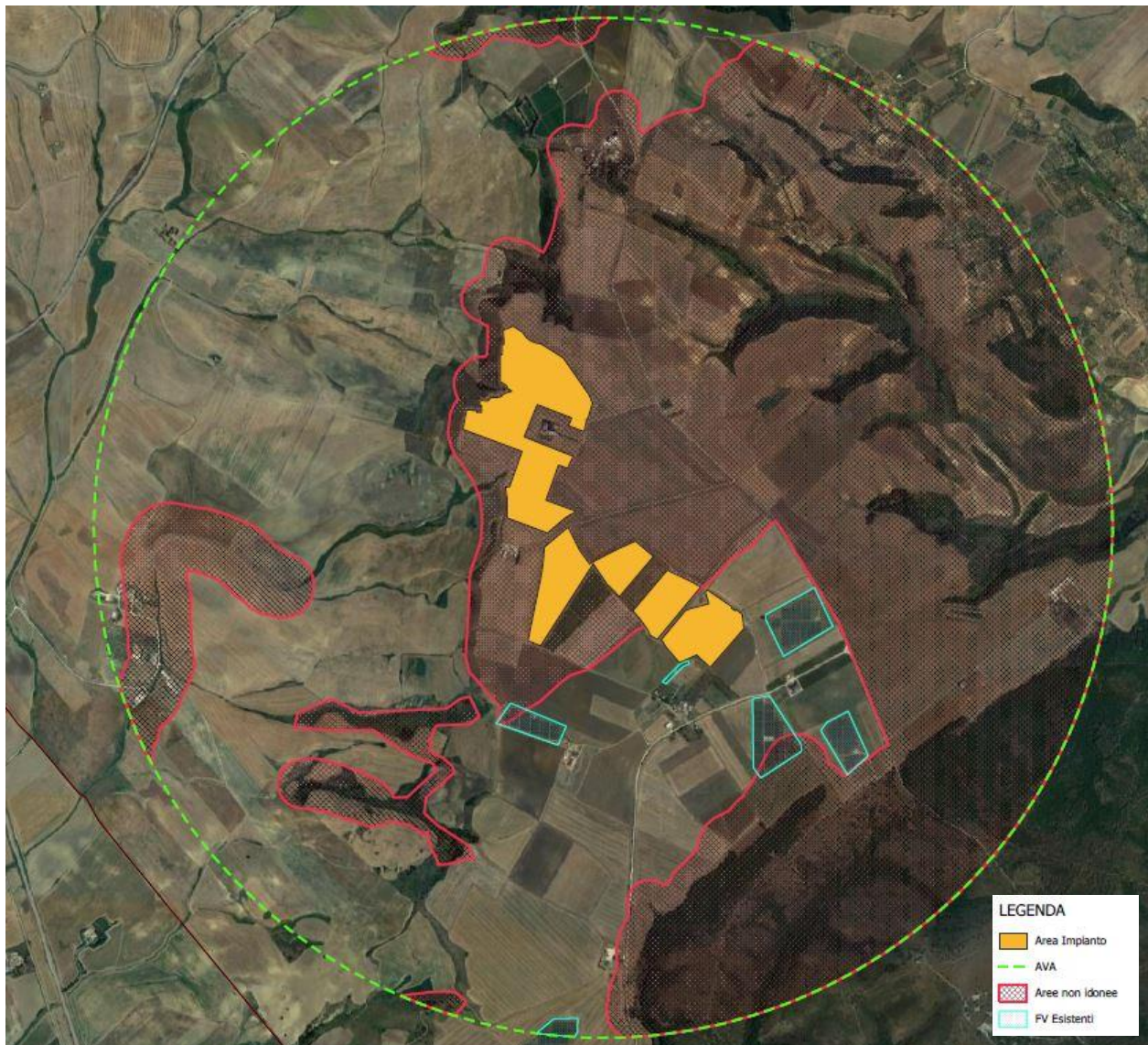
Figura 16-35: Area di Valutazione Ambientale e FER autorizzati all'interno dell'AVA
