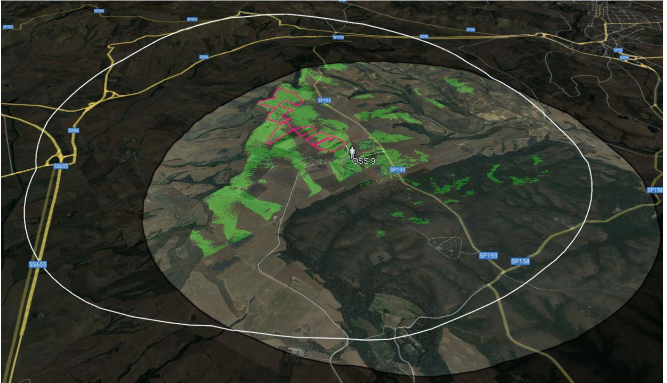
Figura 16-29: OSSERVATORE 9: Area di visibilità teorica
