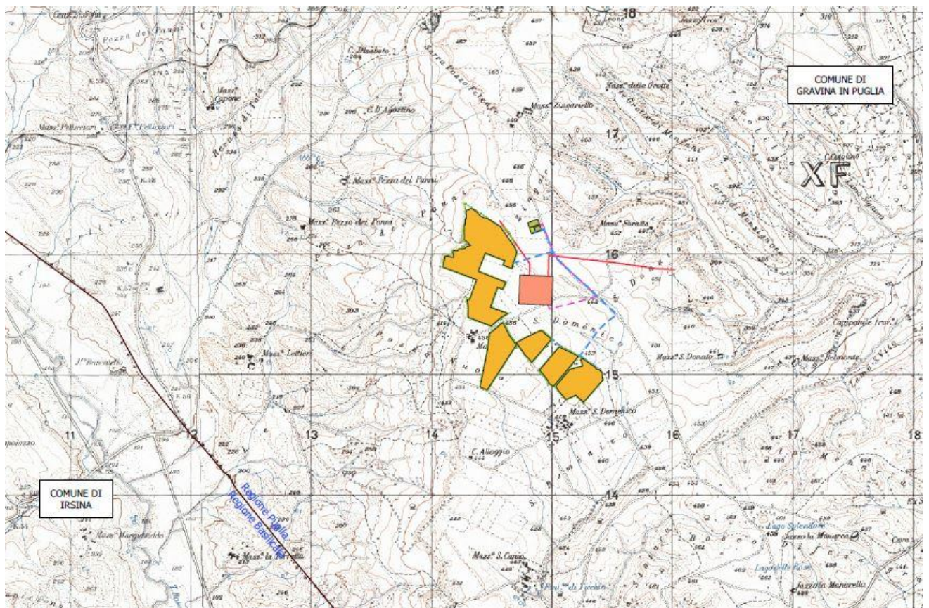
Figura 9-1: Inquadramento layout di impianto su base IGM
