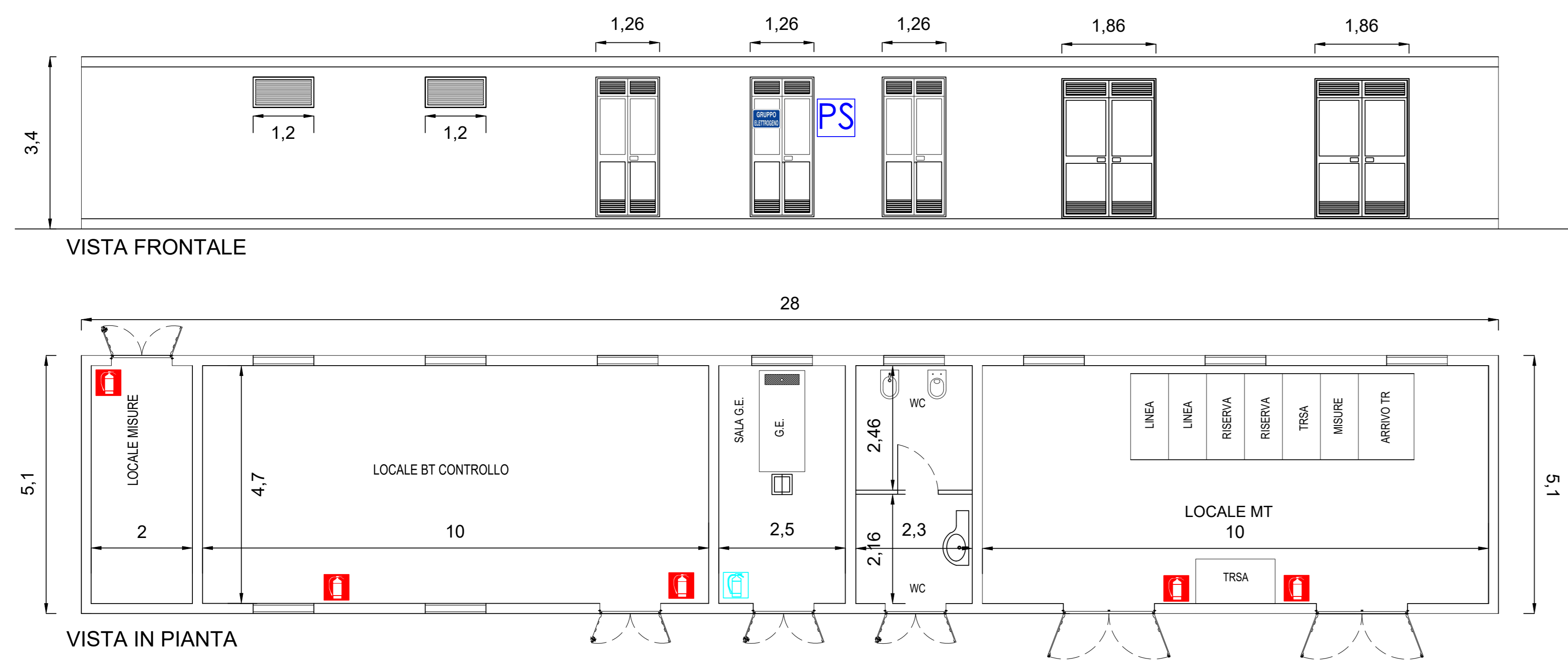
Planimetria edificio di controllo della stazione - Scala 1:75
