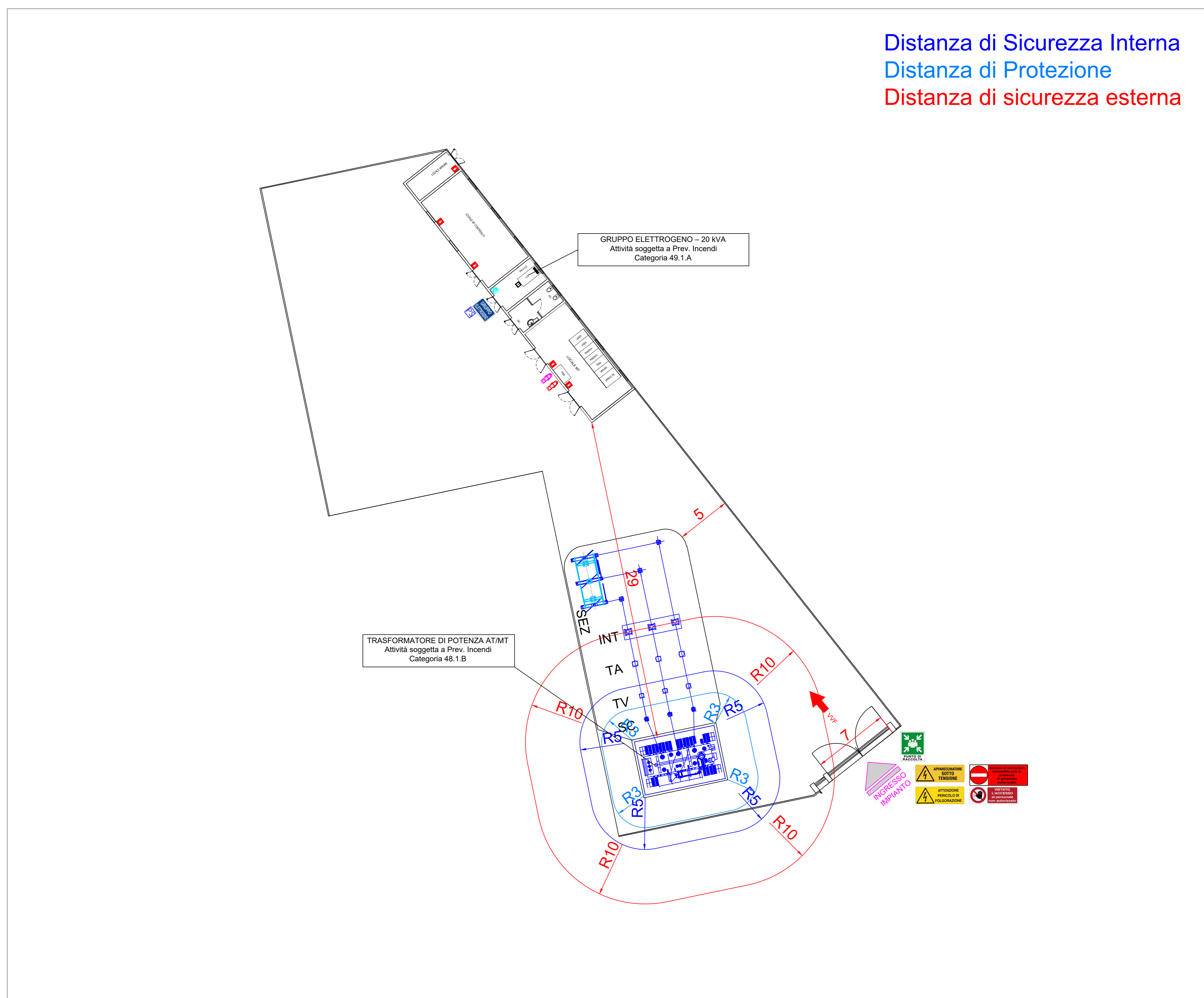
Planimetria sottostazione di progetto, distanze di sicurezza esterne, interne e di protezione - Scala 1:200
