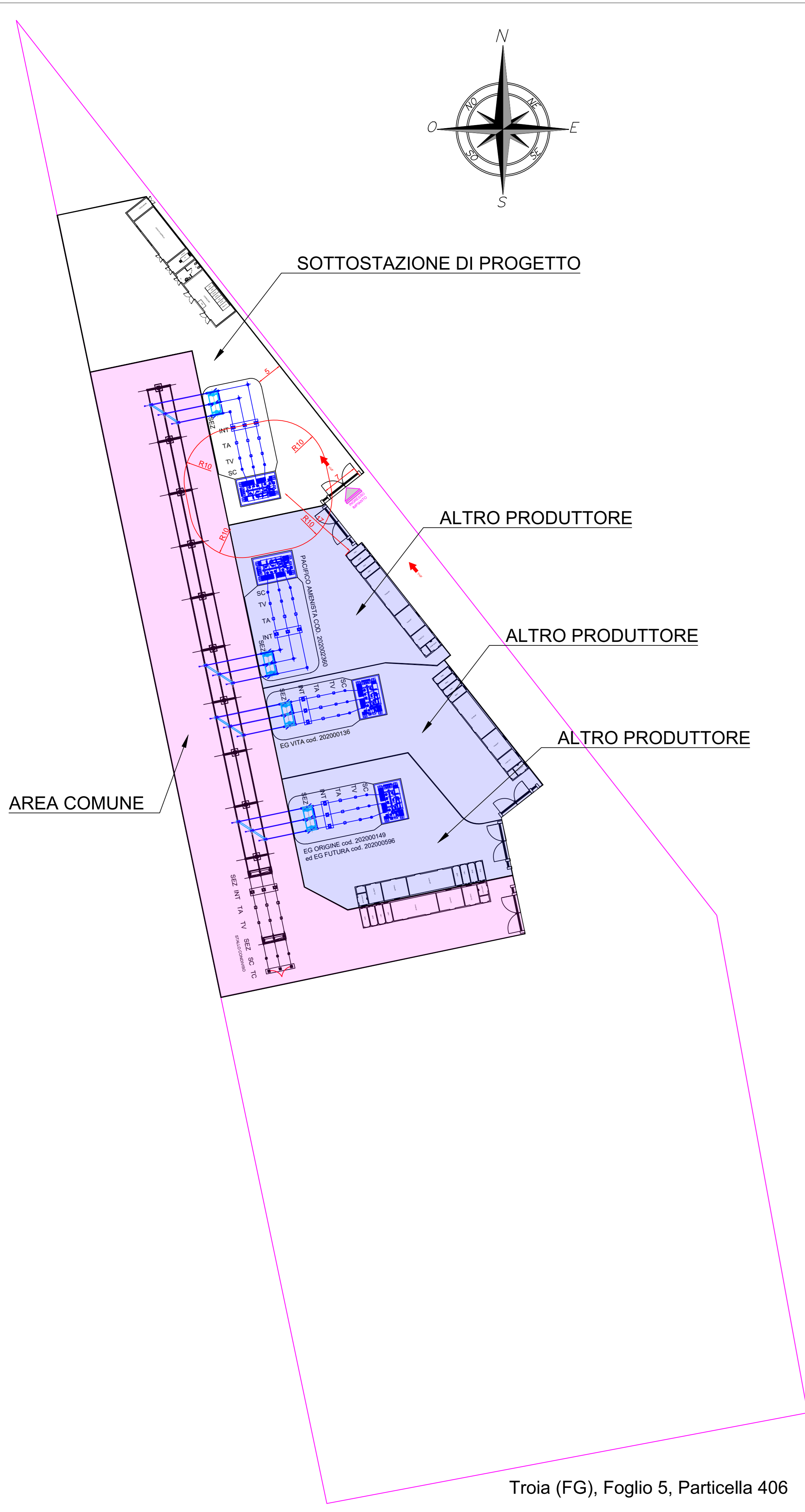
Planimetria sottostazione distanze di sicurezza esterne - Scala 1:500
