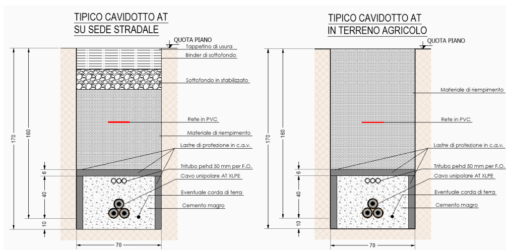
Figura 14: Esempio tipologico scavo AT
