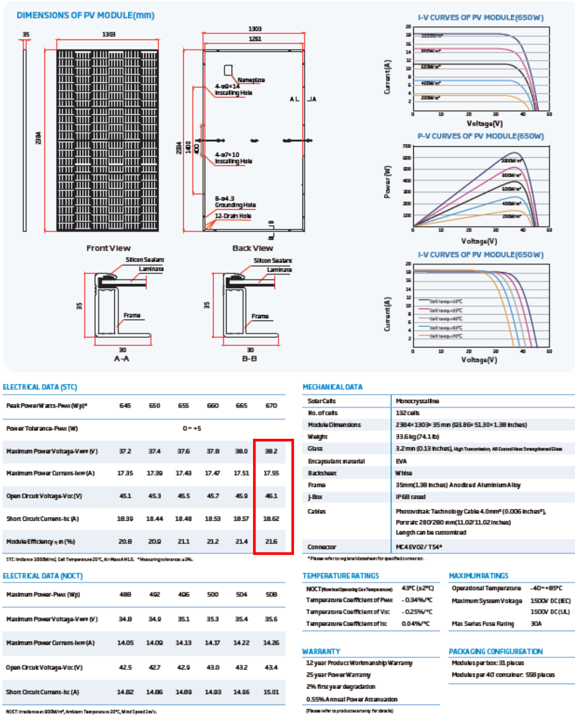
Figura 1: Scheda tecnica del modulo fotovoltaico
