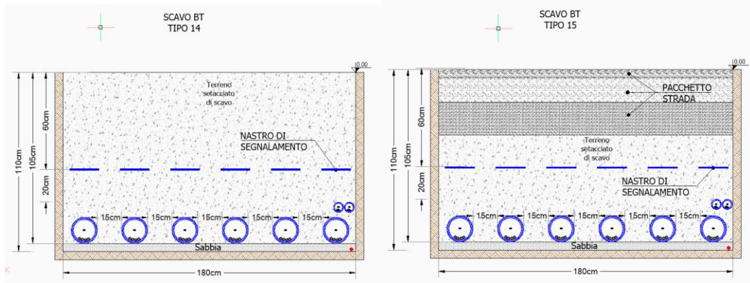
Figura 12: Esempi tipici scavo BT
