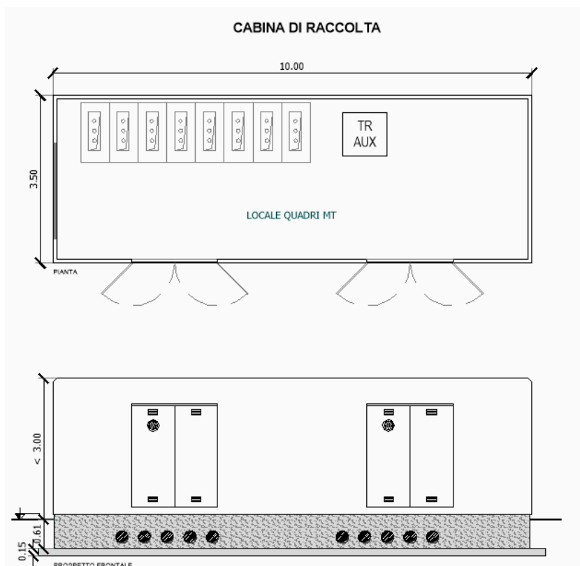
Figura 10: Prospetto di una cabina di raccolta
