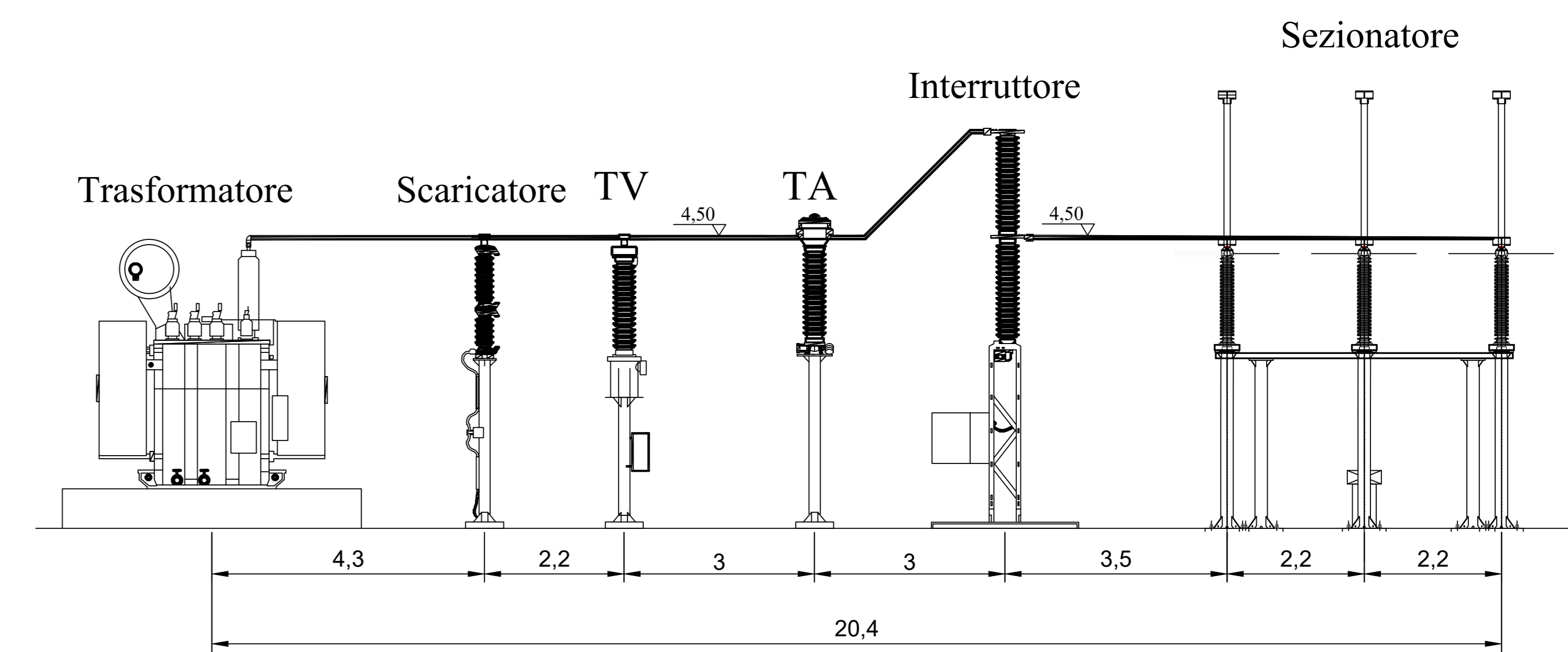
Sezione B-B'
