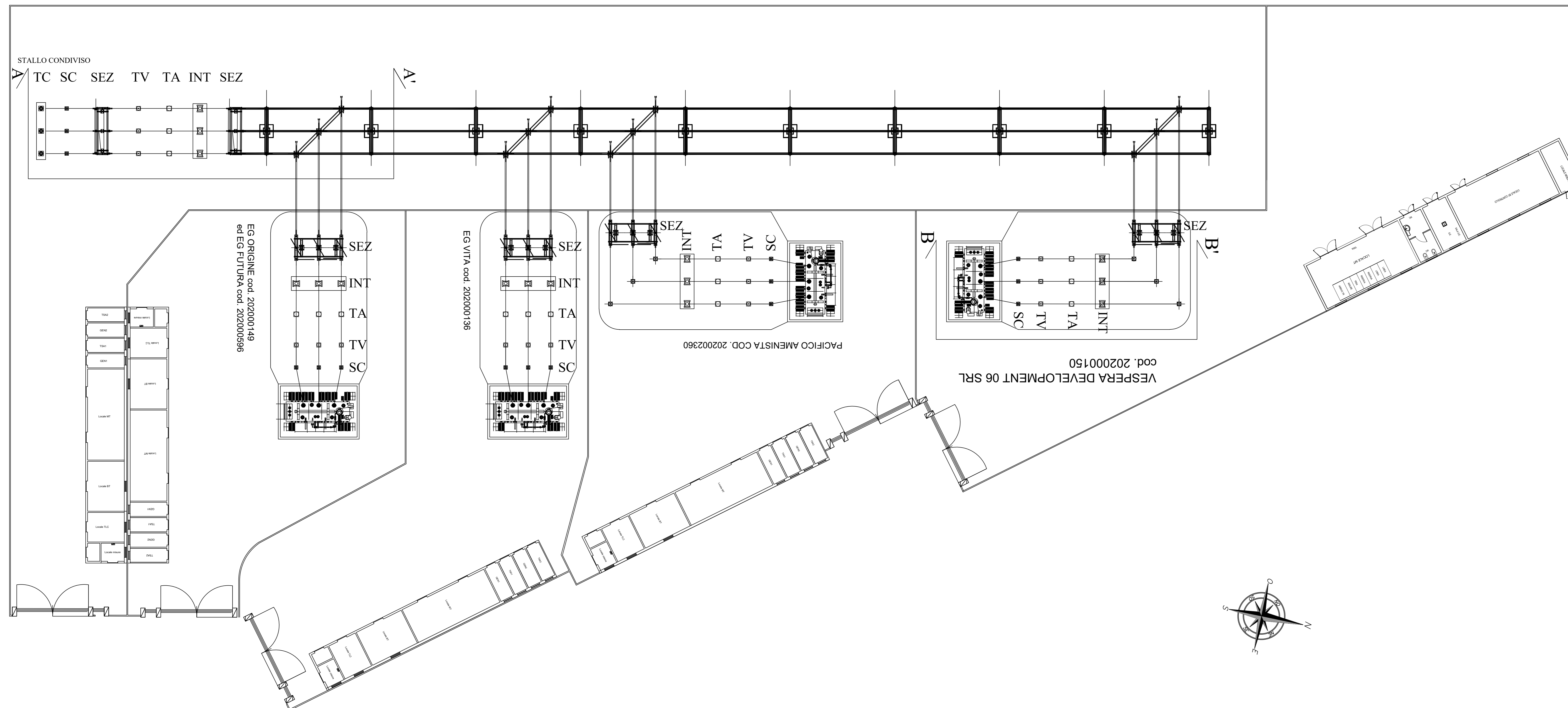
Planimetria Sottostazione Utente AT/MT e sezioni elettromeccaniche - Non in scala
