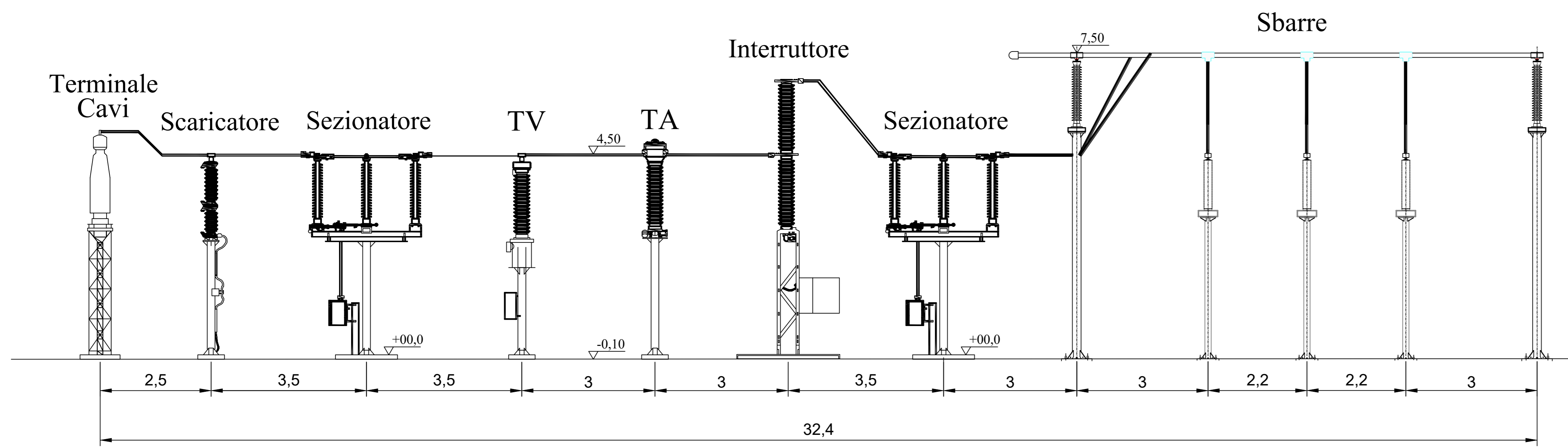
Sezione A-A'
