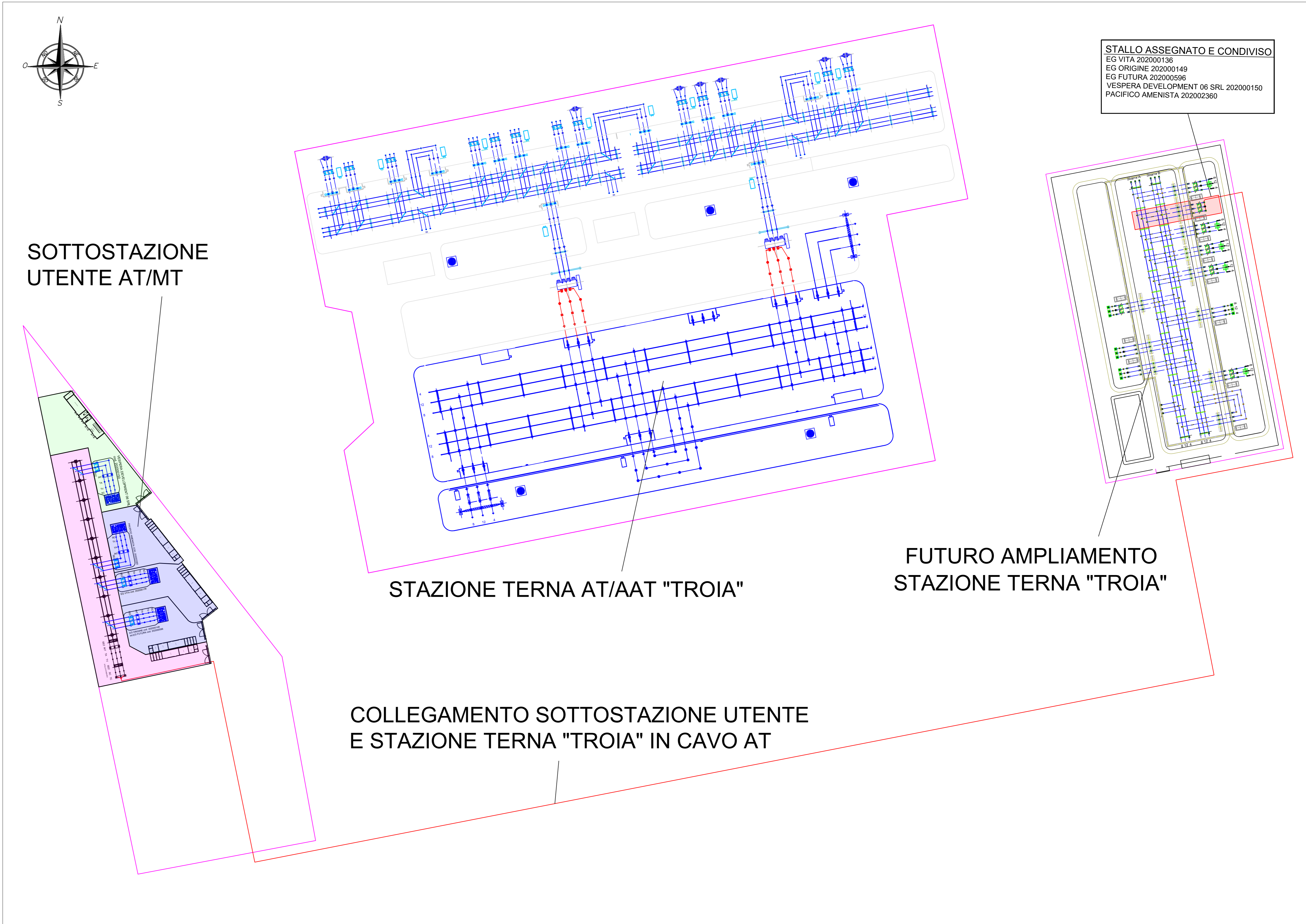
Planimetria Sottostazione Utente AT/MT e Stazione AT/AAT "Troia" - Scala 1:1000
