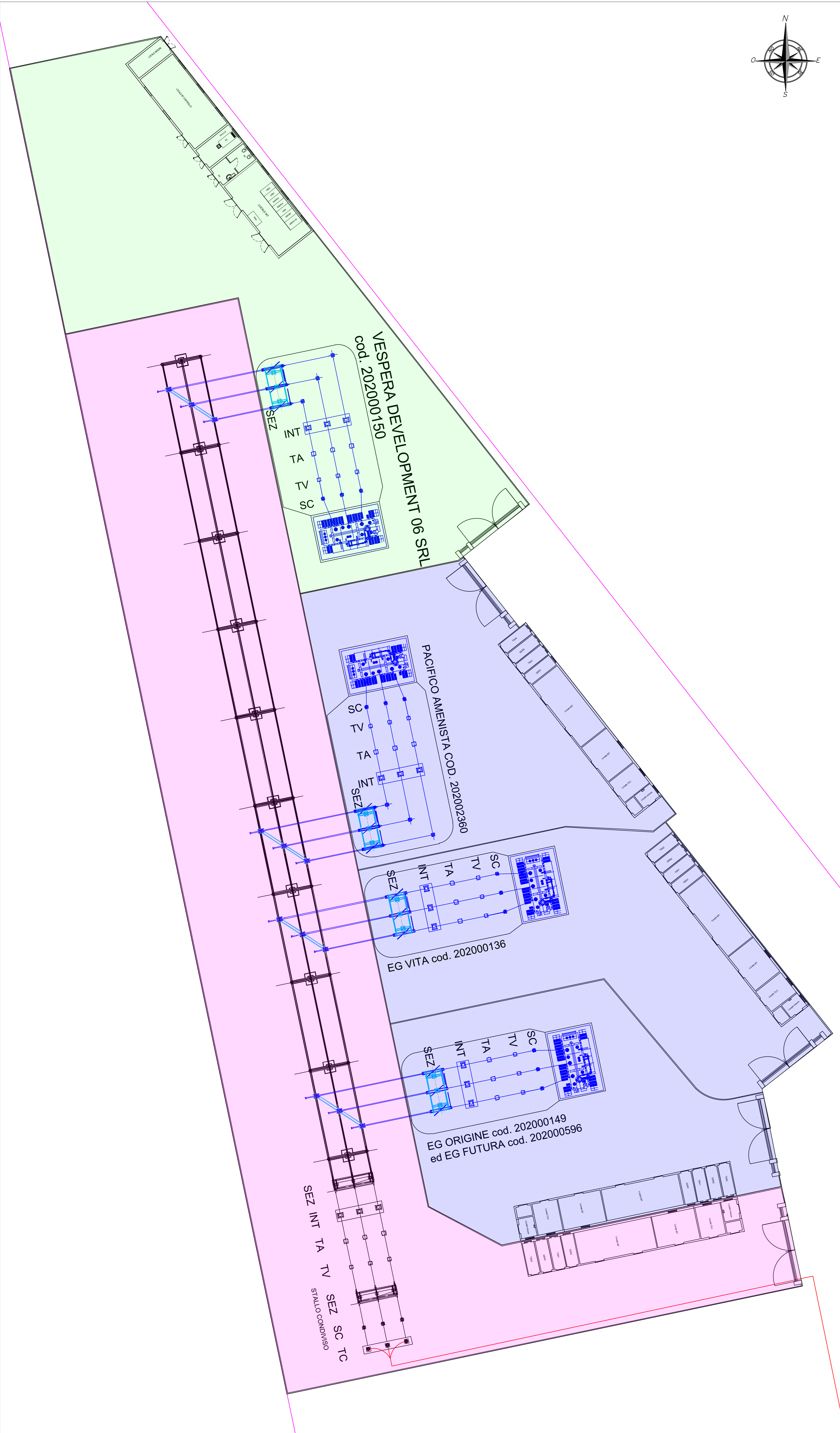
Planimetria Sottostazione Utente AT/MT- Scala 1:200
