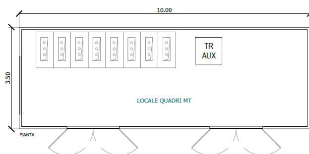
Figura 24: Pianta cabina di raccolta
