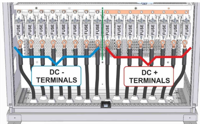
Figura 38: Connessione dei cavi provenienti dalle string-box alla sezione d'ingresso dell'inverter centralizzato scelto
