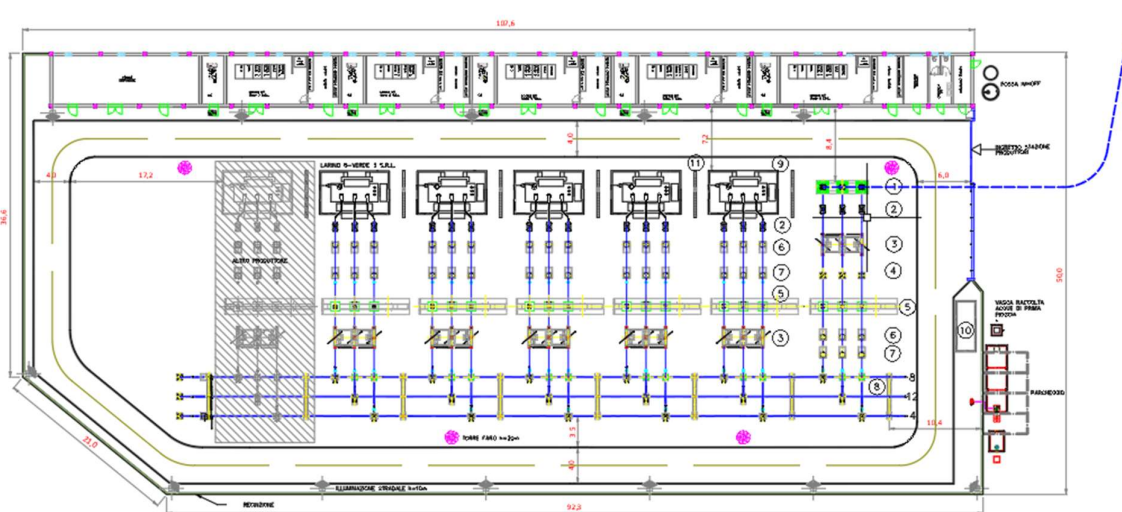
Schema grafico dei componenti dell’Impianto di Utenza
