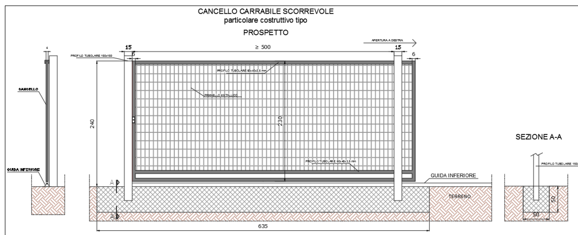
Figura 18 – CANCELLO carrabile scorrevole - Particolare costruttivo
