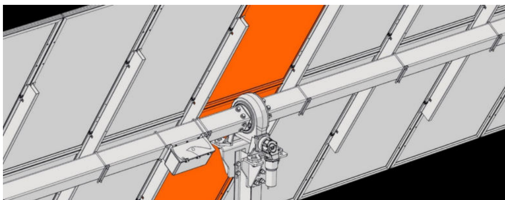
Figura 17 A – Particolare dell'inseguitore installato
