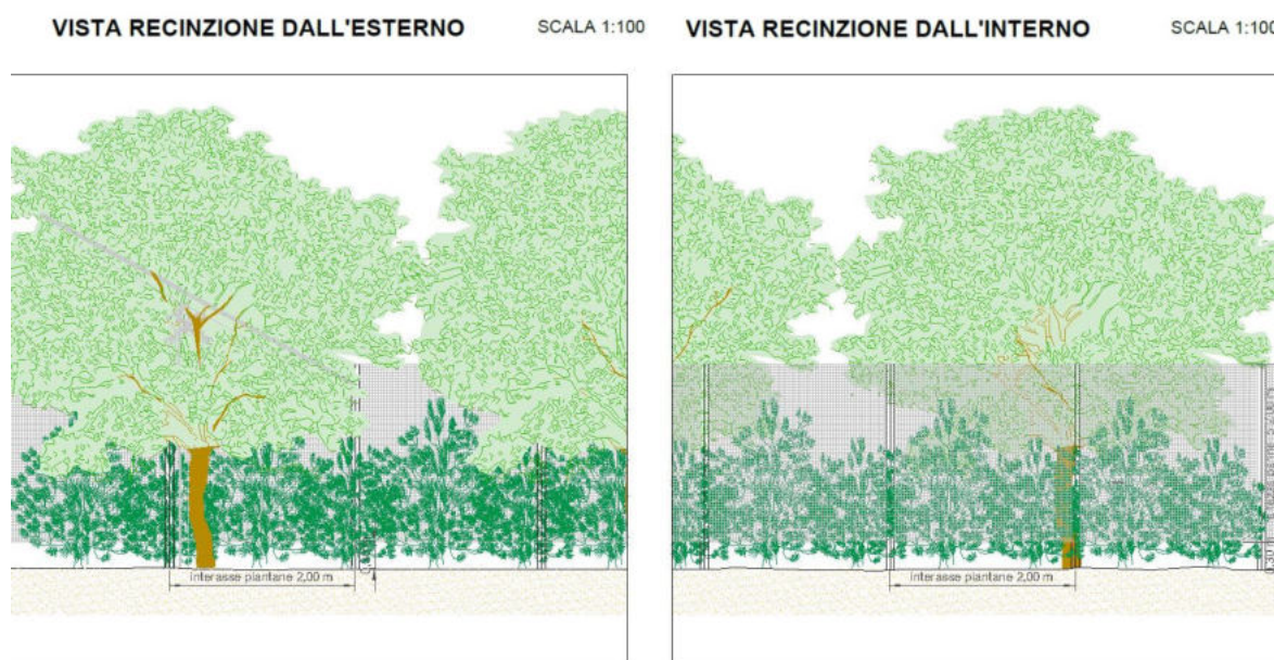
Fig. 10 - Dettaglio della recinzione dell'impianto agro-fotovoltaico
