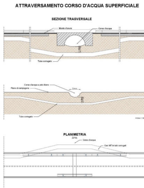
Figura 22 – Particolare attraversamento corso d'acqua superficiale e tipologia di attraversamento su strada
