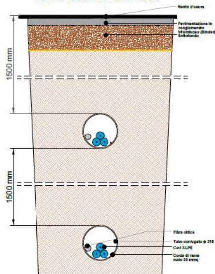
Figura 31 B – Particolare sezione tipo cavo AT
