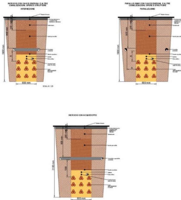
Fig. 31 A – Sezione tipo-posa cavi MT
