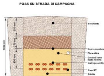
Figura 19 – Particolare sezione tipo cavo interrato BT
