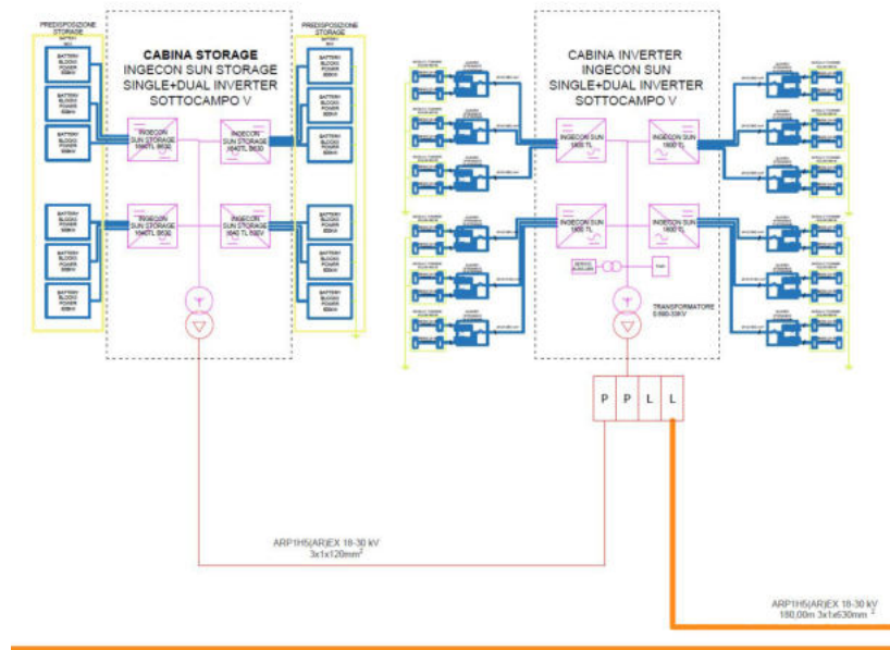
Schema elettrico (TAV. IT-SEU)
