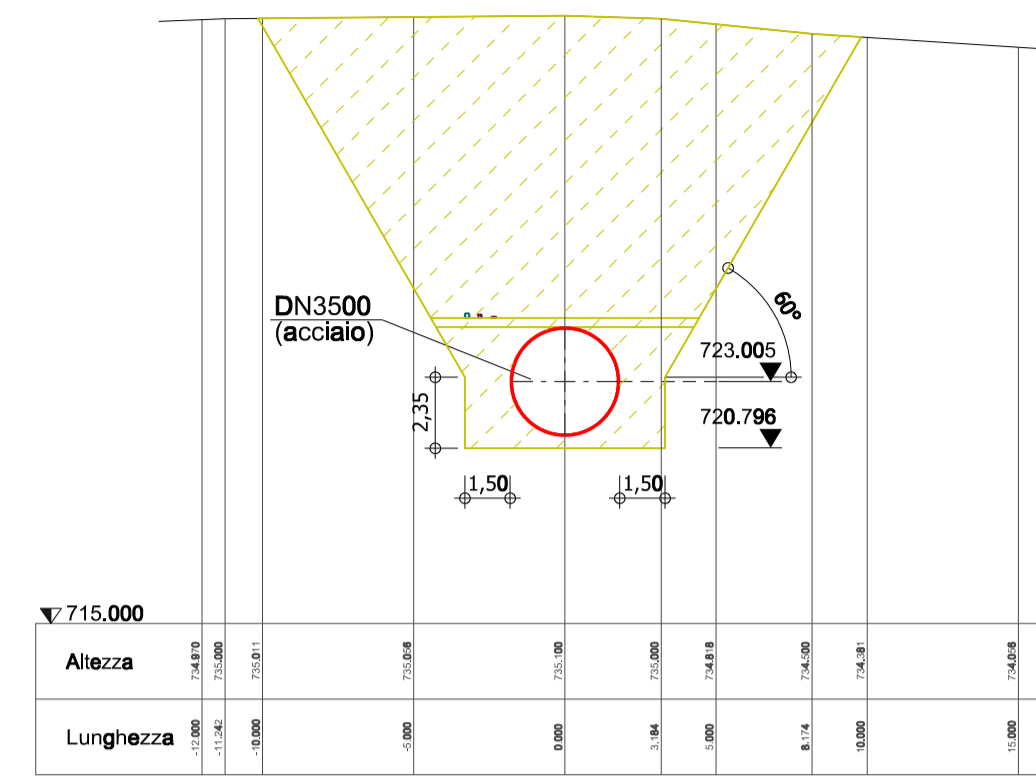
Sezione: 3+200 Scala 1:250
