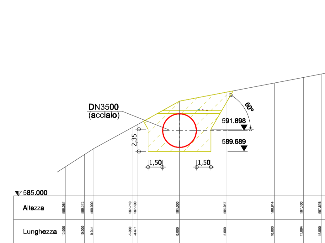
Sezione: 3+900 Scala 1:250
