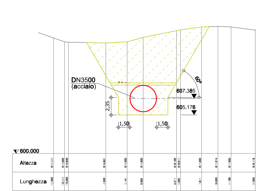
Sezione: 3+600 Scala 1:250
