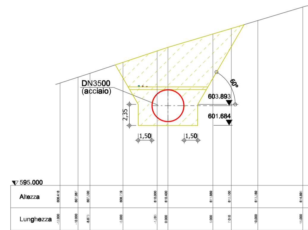
Sezione: 3+700 Scala 1:250
