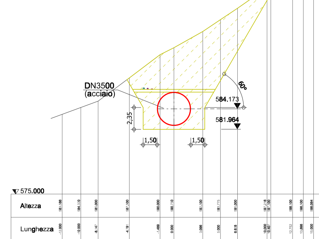
Sezione: 4+200 Scala 1:250
