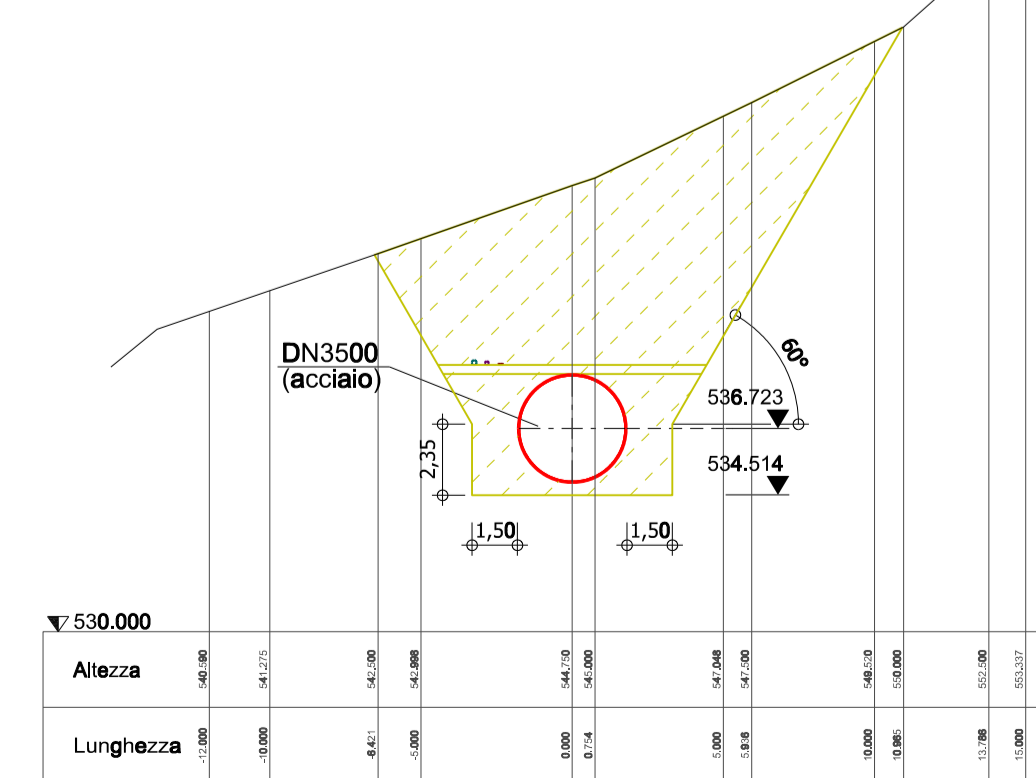
Sezione: 4+400 Scala 1:250
