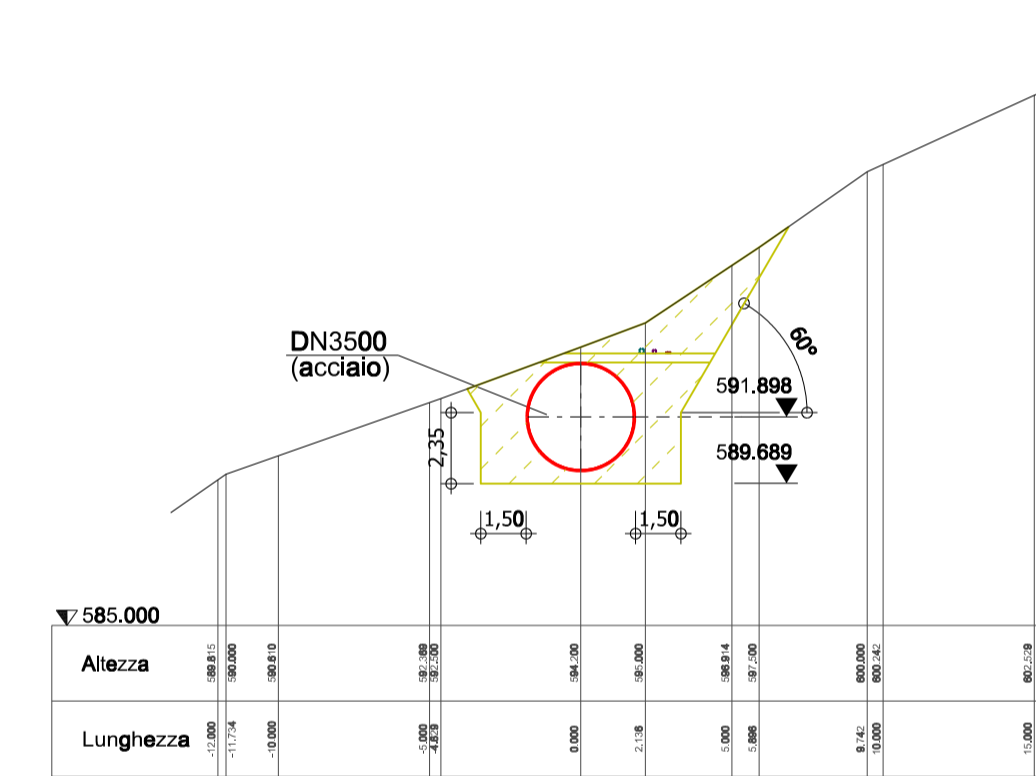
Sezione: 4+000 Scala 1:250
