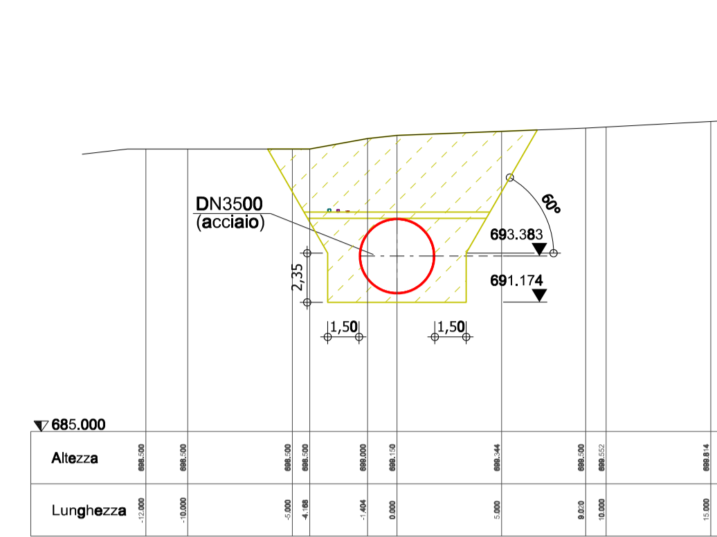
Sezione: 3+300 Scala 1:250
