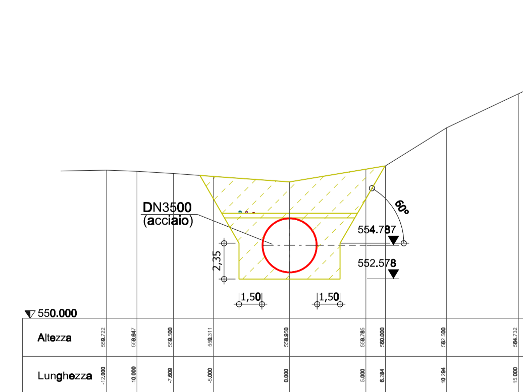
Sezione: 4+300 Scala 1:250
