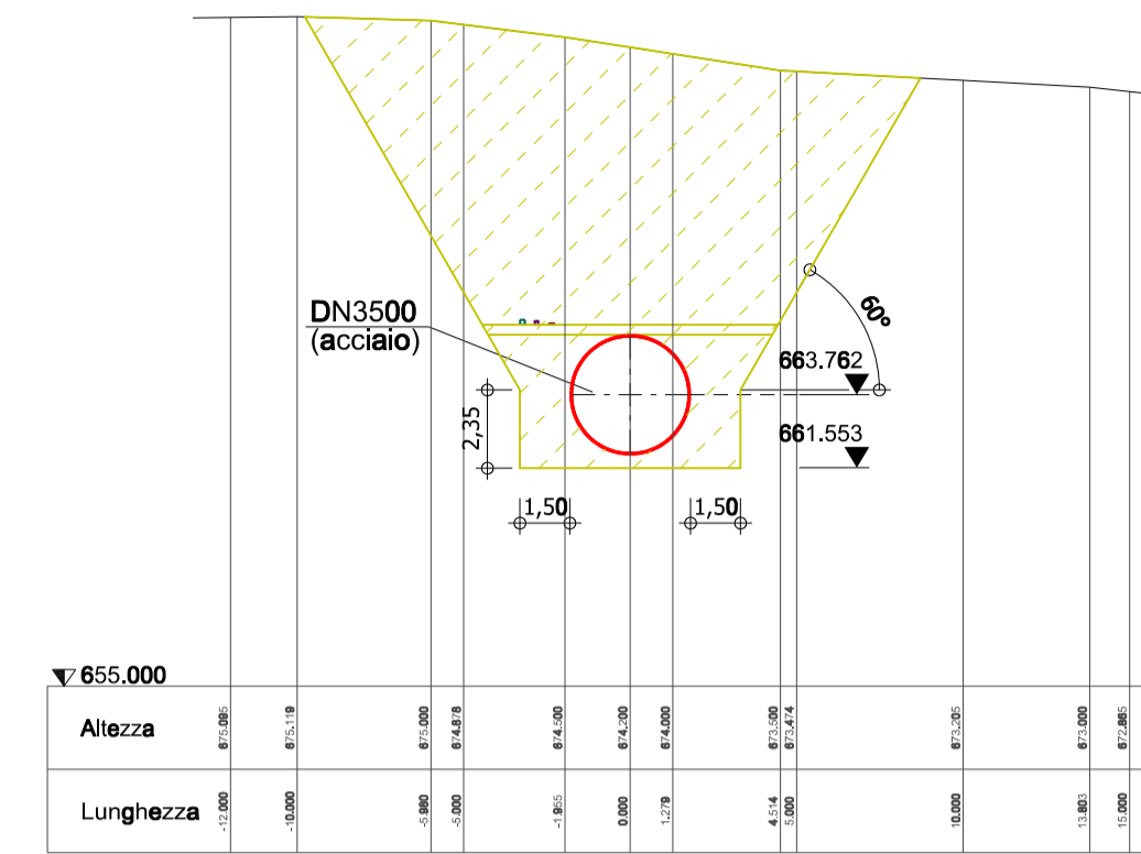
Sezione: 3+400 Scala 1:250
