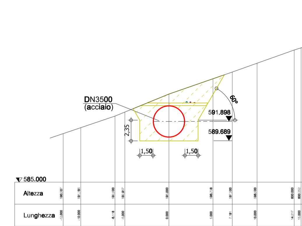
Sezione: 4+100 Scala 1:250
