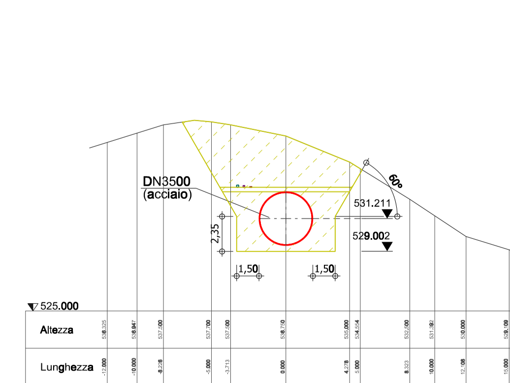
Sezione: 4+500 Scala 1:250
