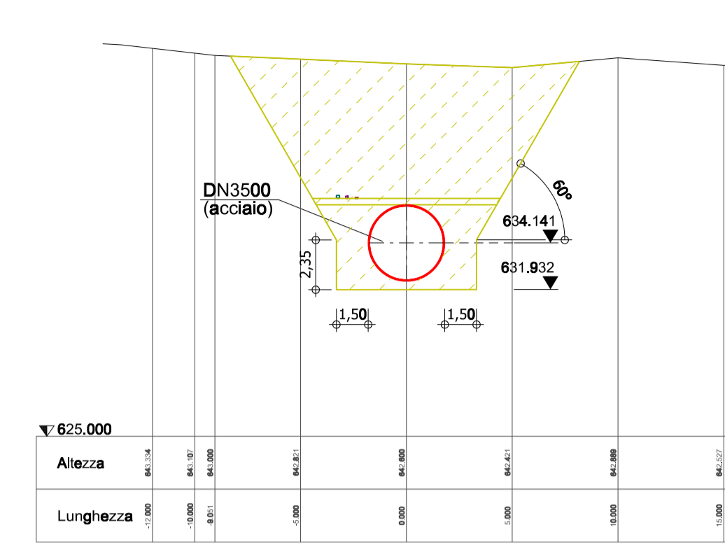
Sezione: 3+500 Scala 1:250
