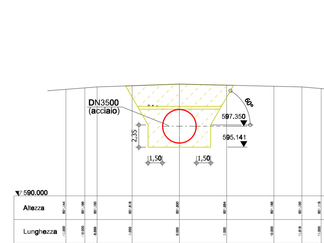
Sezione: 3+800 Scala 1:250
