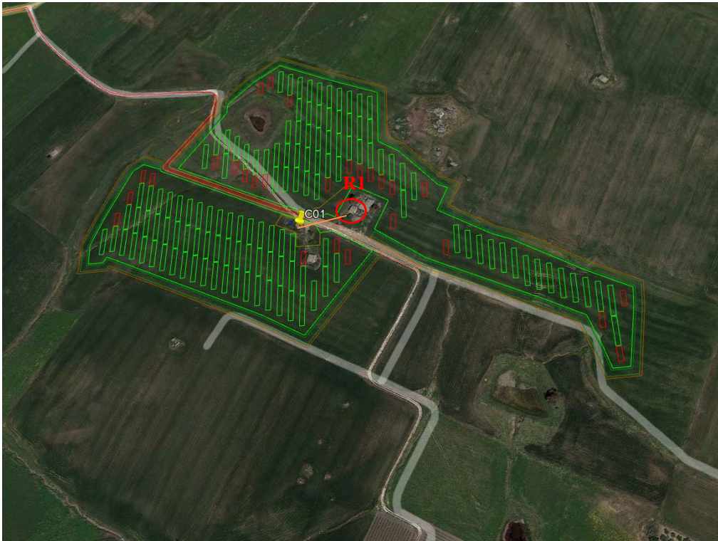
IMPIANTO AREA NORD: INDIVIDUAZIONE DEL RICETTORE R1 RISPETTO ALLA POWER STATION
