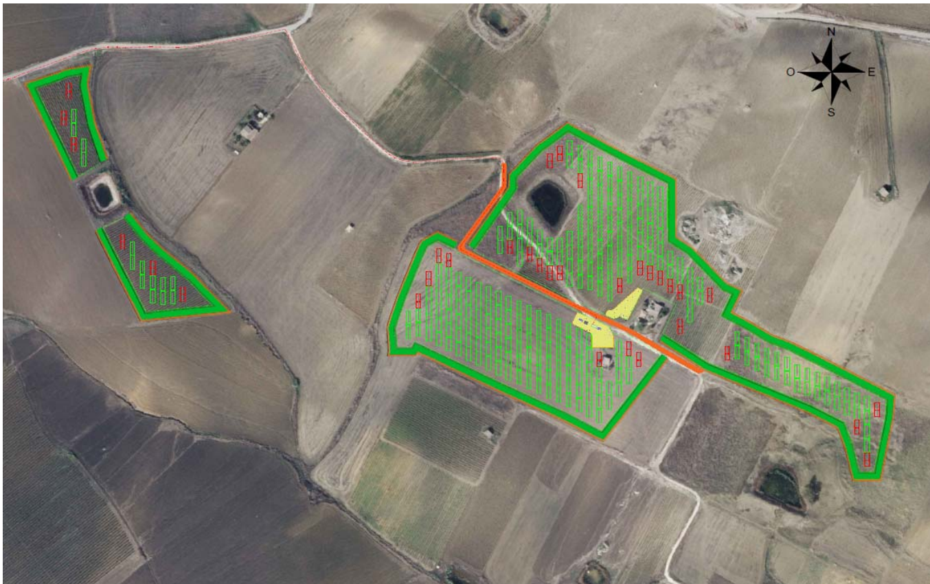
LAYOUT IMPIANTO AREA NORD
