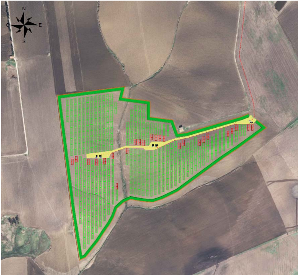
LAYOUT IMPIANTO AREA SUD
