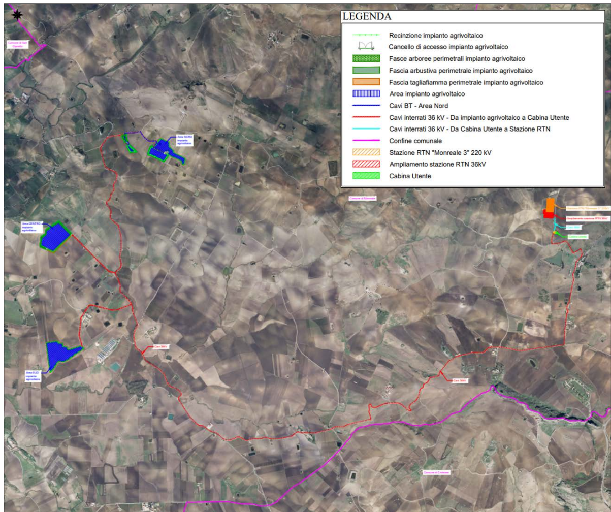
Figura 4 – Stralcio Ortofotocarta impianto agrivoltaico
