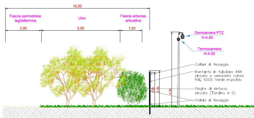
Fascia di mitigazione rispetto alla recinzione
