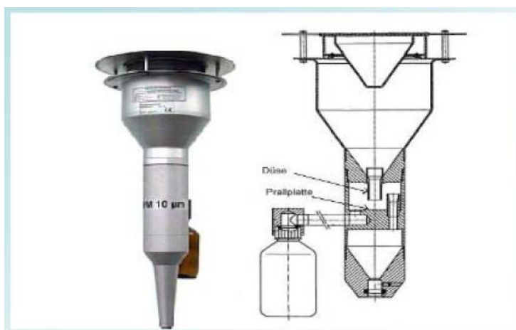
Testa di campionamento per il prelievo del particolato
