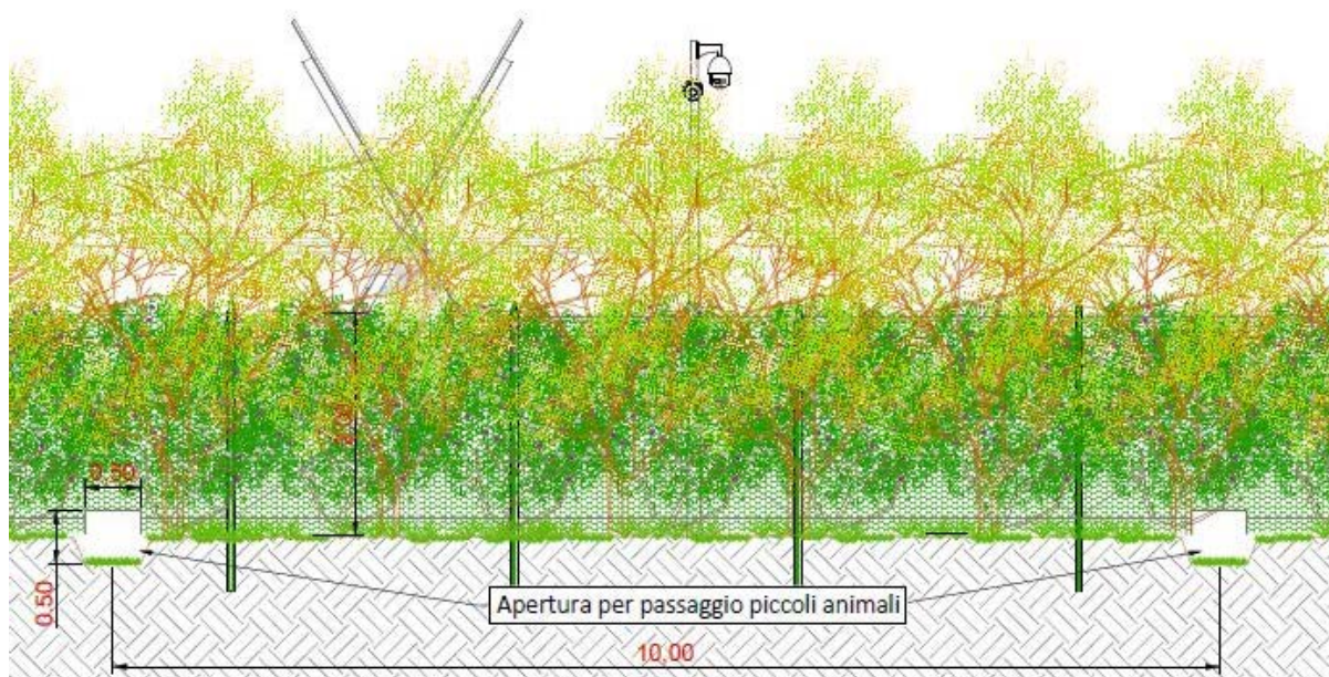
Particolari aperture per il passaggio della fauna in corrispondenza della recinzione perimetrale
