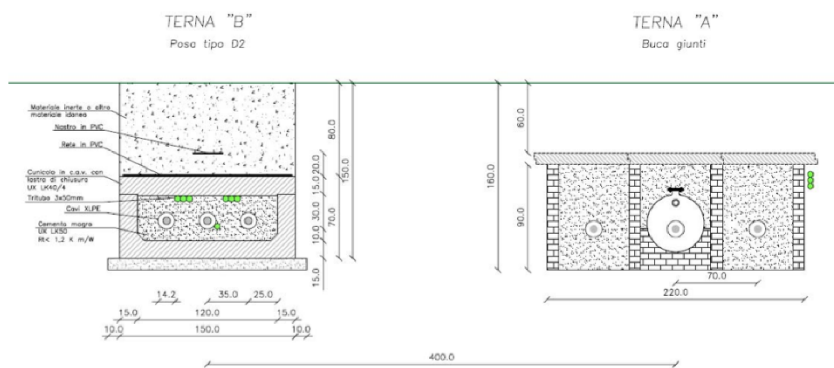
Figura 2: Affiancamento tra due linee interrate AT
