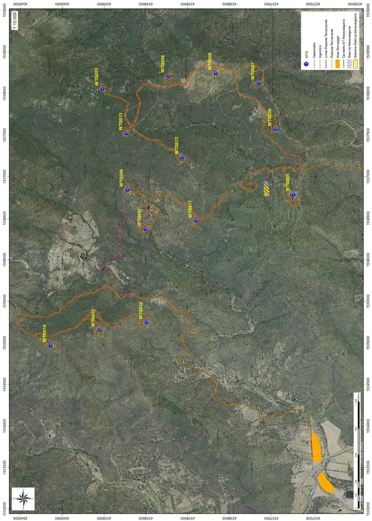
Figura 1 - Layout di impianto e viabilità interna
