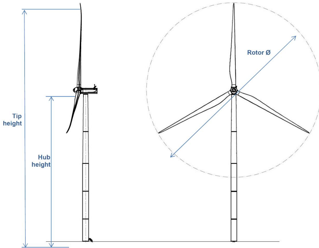
Figura 2—generatore eolico ad asse orizzontale
