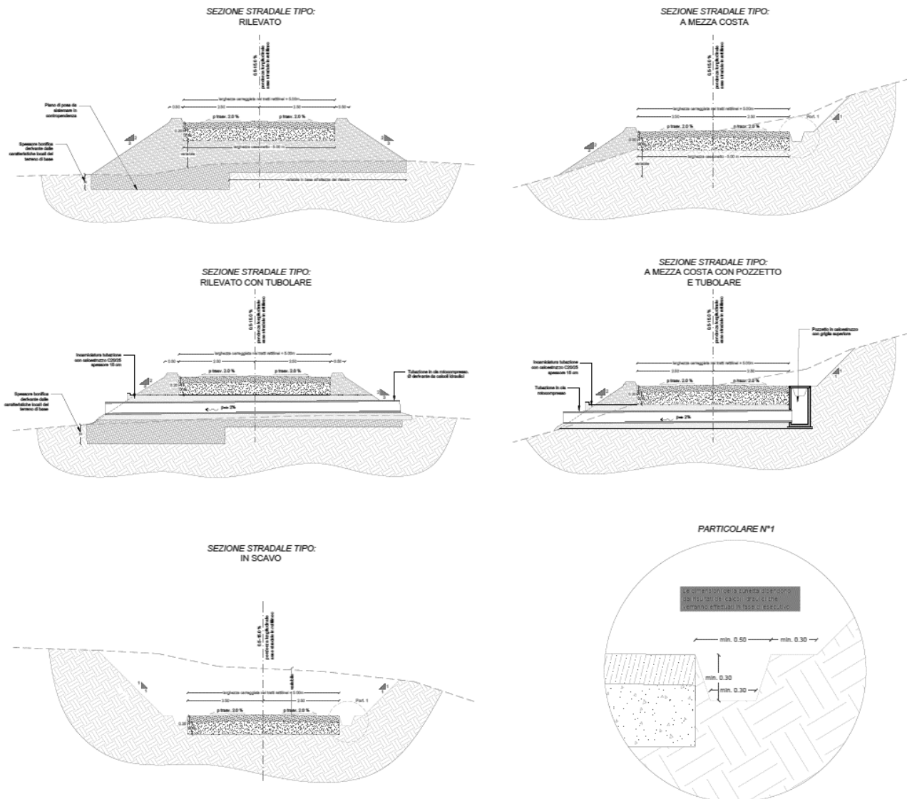
Figura 3- Sezioni tipo viabilità interna al parco
