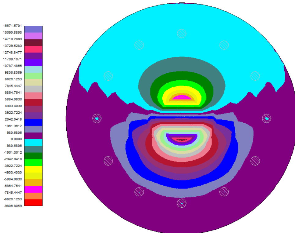
Momenti M_y
