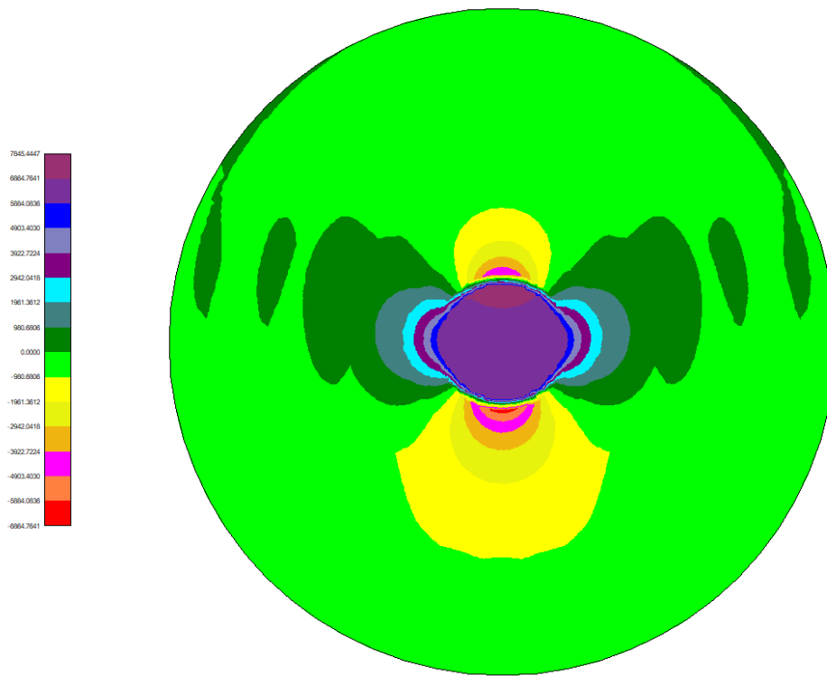
Diagramma del taglio T_y
