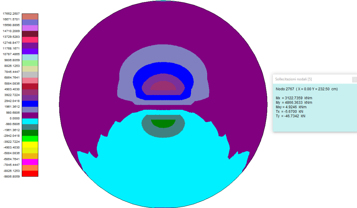
Sollecitazioni da carico medio, punto di coordinate (0;+232.5)
