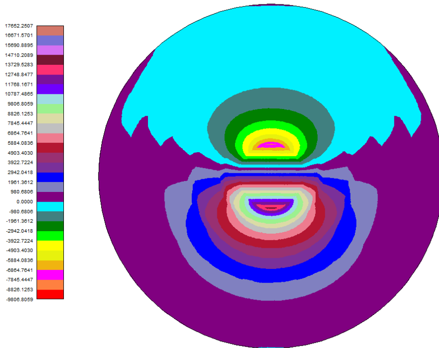
Momenti M_y
