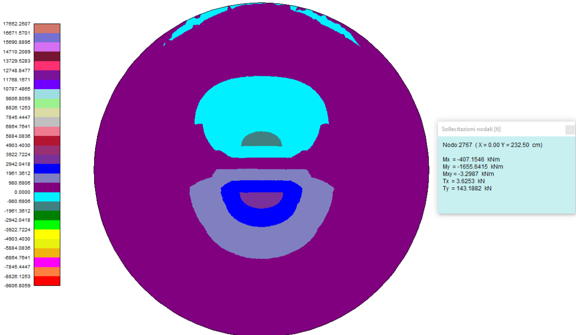
Sollecitazioni per range m=7, punto di coordinate (0;+232.5)
