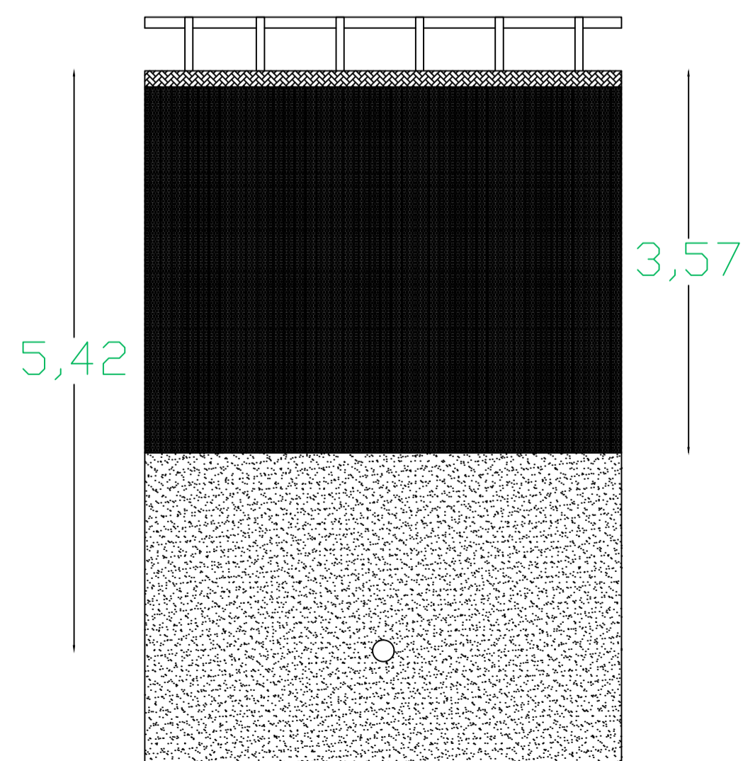
SEZIONE 2
