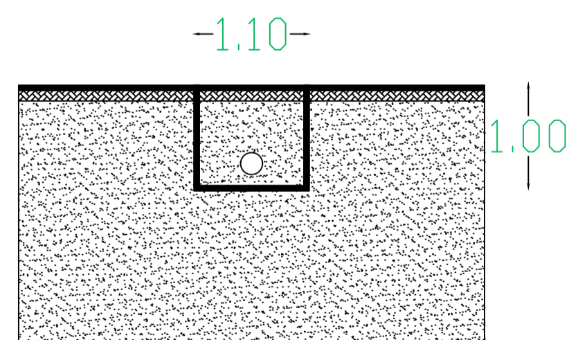
SEZIONE 1 = SEZIONE 3
