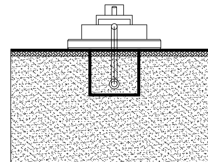
SEZIONE 4
