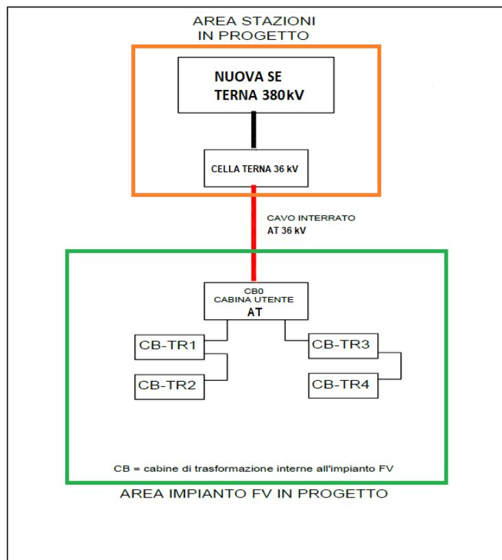
FIGURA 5: SCHEMA A BLOCCHI IMPIANTO
