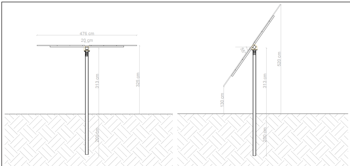
FIGURA 1: TRACKER SOLARE TIPO
