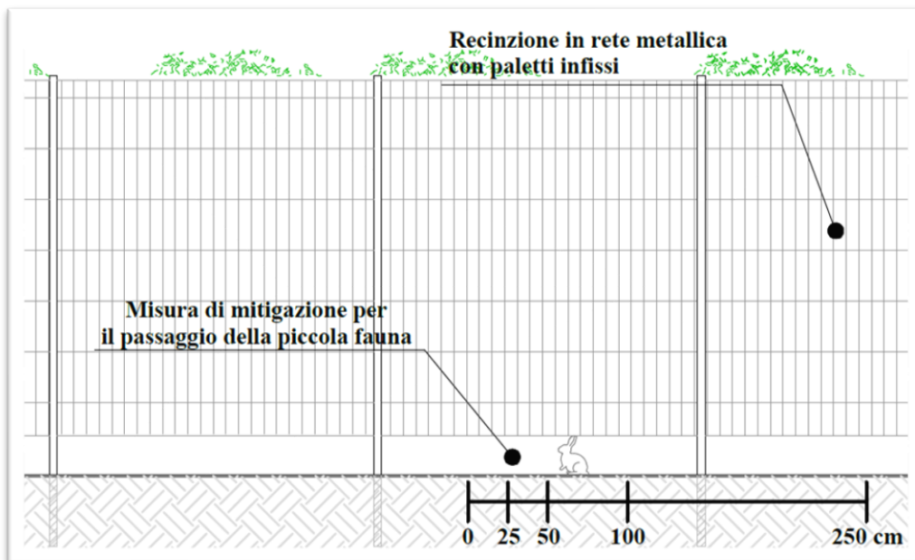
FIGURA 9: RECINZIONE TIPO
