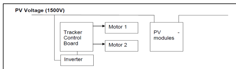
FIGURA 5: ALIMENTAZIONE DEL MOTORE DEI TRACKER DIRETTAMENTE DAL CAMPO FV
