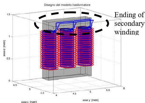
Fig. 14: Connessioni elettriche considerate al lati BT.
