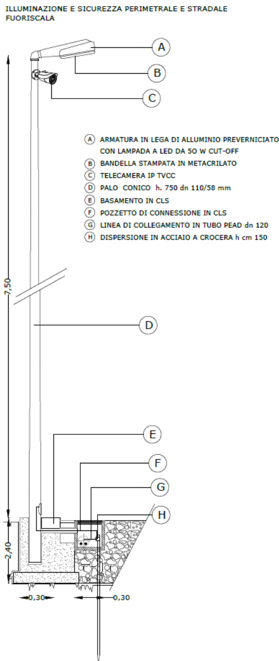
FIGURA 35 – ESEMPIO IMPIANTO DI ILLUMINAZIONE INTEGRATO CON SISTEMA DI VIDEOSORVEGLIANZA – ESTRATTO DALL'ELABORATO TECNICO PLOGAGHE-PDR02
