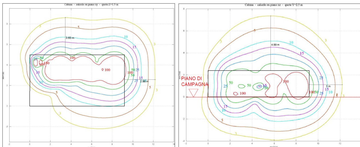
FIGURA 78 – CURVE ISOINDUZIONE AT/BT CABINA DI SOTTOCAMPO – VISTA IN PIANTA (A SX) E PROSPETTO (A DX). STRALCIO DELL'ELABORATO PLOAGHE-PDT13
