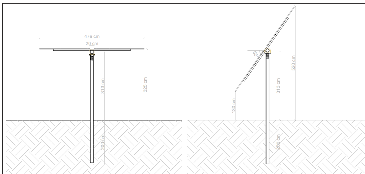
FIGURA 29 – TRACKER TIPO AD ASSE VARIABILE
