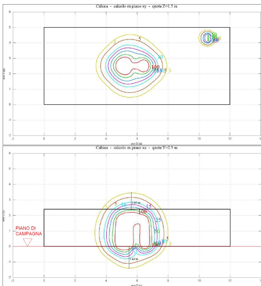
FIGURA 79 – CURVE ISOINDUZIONE CABINA AT CONSEGNA – PIANTE (IN ALTO) E PROSPETTO FRONTALE (IN BASSO). STRALCIO DELL'ELABORATO PLOAGHE-PDT13.
