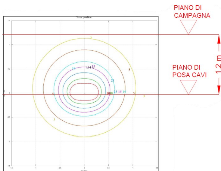
FIGURA 76 – CURVE ISOINDUZIONE – 3 LINEE BT INTERRATE (STRALCIO DELL'ELABORATO CARTOGRAFICO PLOAGHE-PDT13)
