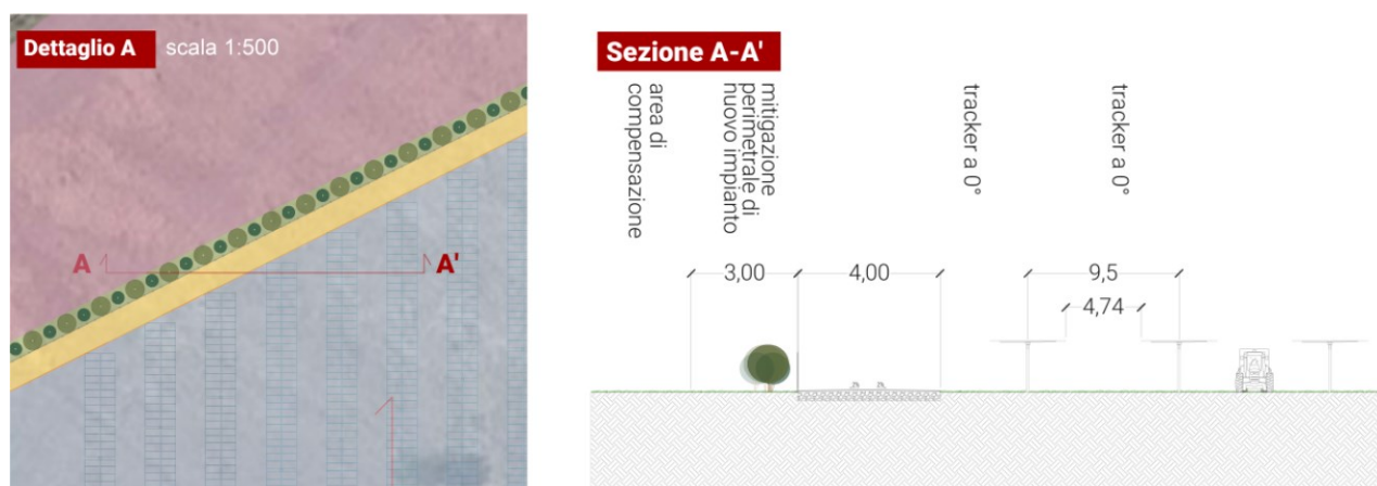
FIGURA 63 – PARTICOLARE FASCIA DI MITIGAZIONE DI NUOVO IMPIANTO E VIABILITÀ PERIMETRALE - SEZIONE O-E DELL'IMPIANTO (ESTRATTO DALL'ELABORATO GRAFICO PLOAGHE-PDT11)
