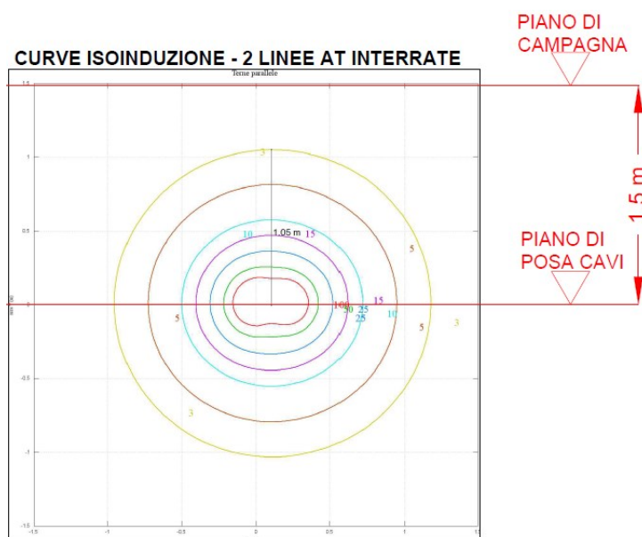
FIGURA 77 – CURVE ISOINDUZIONE – 2 LINEE AT INTERRATE (STRALCIO DELL'ELABORATO CARTOGRAFICO PLOAGHE-PDT13)
