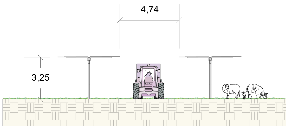
FIGURA 30 – SISTEMA AGRIVOLTAICO ELEVATO, SEZIONE TIPOLOGICA DELL'IMPIANTO
