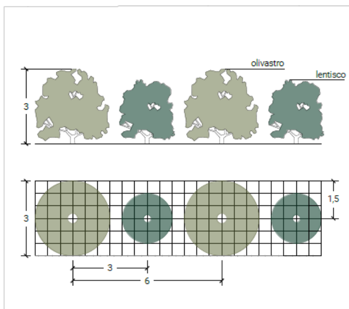
FIGURA 62 – PLANIMETRIA GENERALE SISTEMAZIONE A VERDE OPERE DI MITIGAZIONE E SCHEMA D'IMPIANTO (ESTRATTO DALL'ELABORATO GRAFICO PLOAGHE-PDT11)
