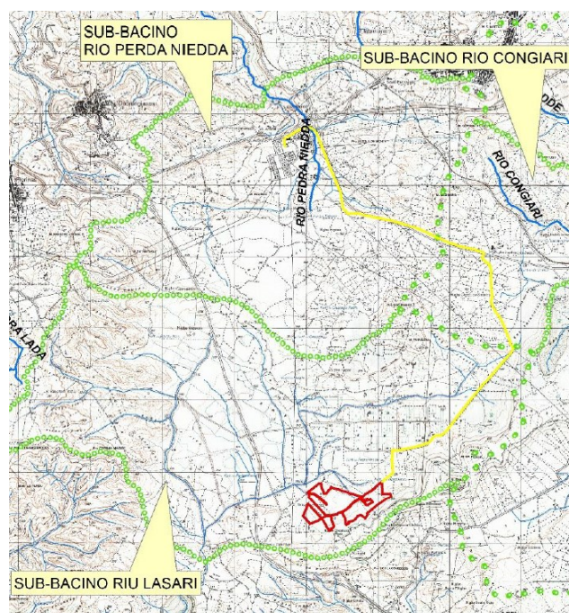
FIGURA 14 – SUDDIVISIONE DELL'AREA DI INDAGINE NEI SUB-BACINI IMBRIFERI DI RIFERIMENTO
