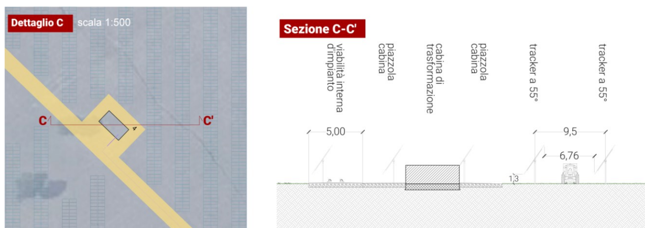
FIGURA 65 – PARTICOLARE AREA CABINA DI TRASFORMAZIONE E RELATIVA SEZIONE N-S DELL'IMPIANTO – ESTRATTO DALL'ELABORATO GRAFICO PLOAGHE-PDT11)
