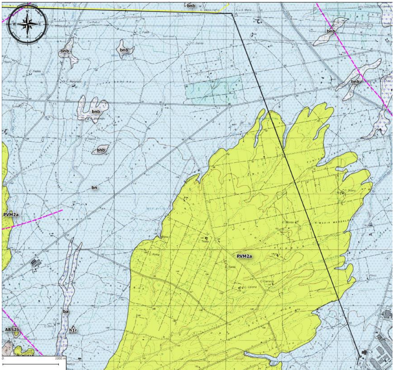
Figura 4 – Estratto della carta geologica
