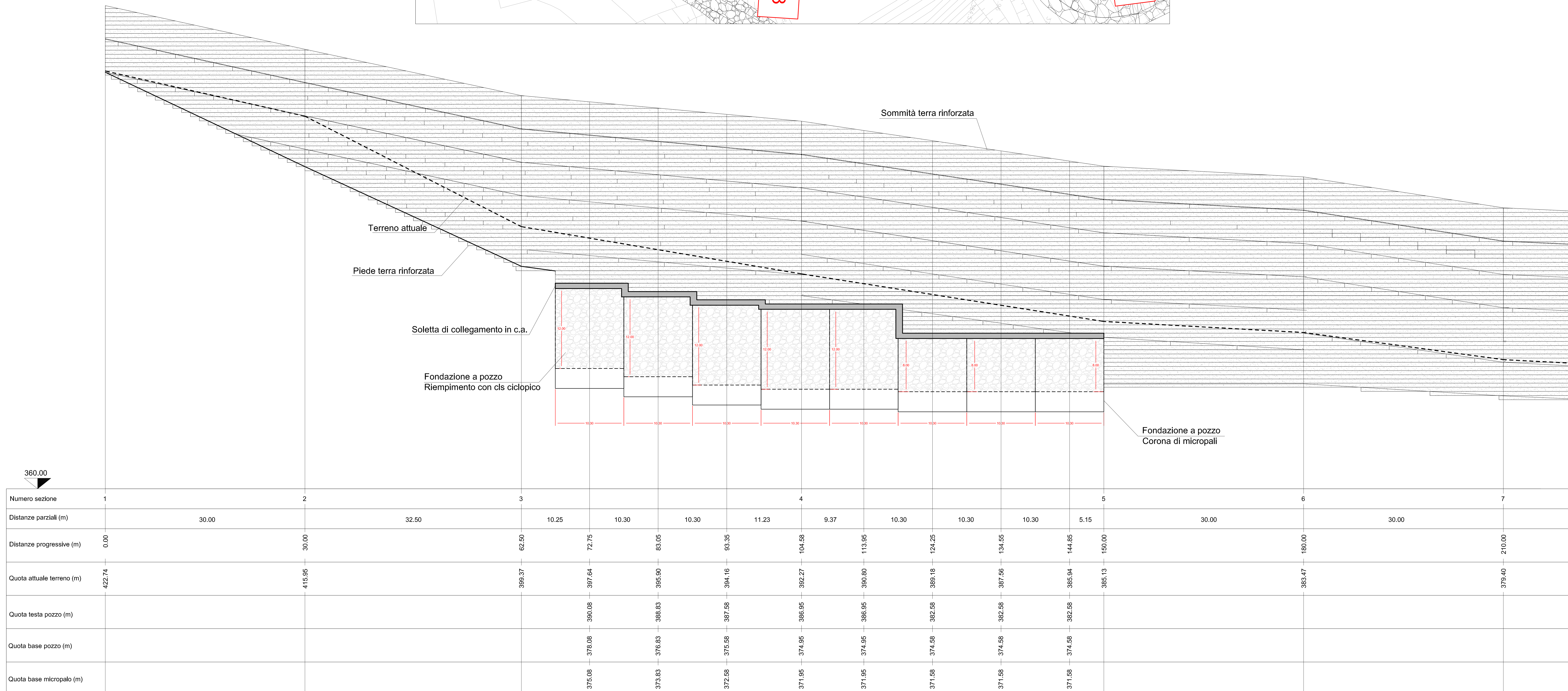
Profilo - scala 1:200
