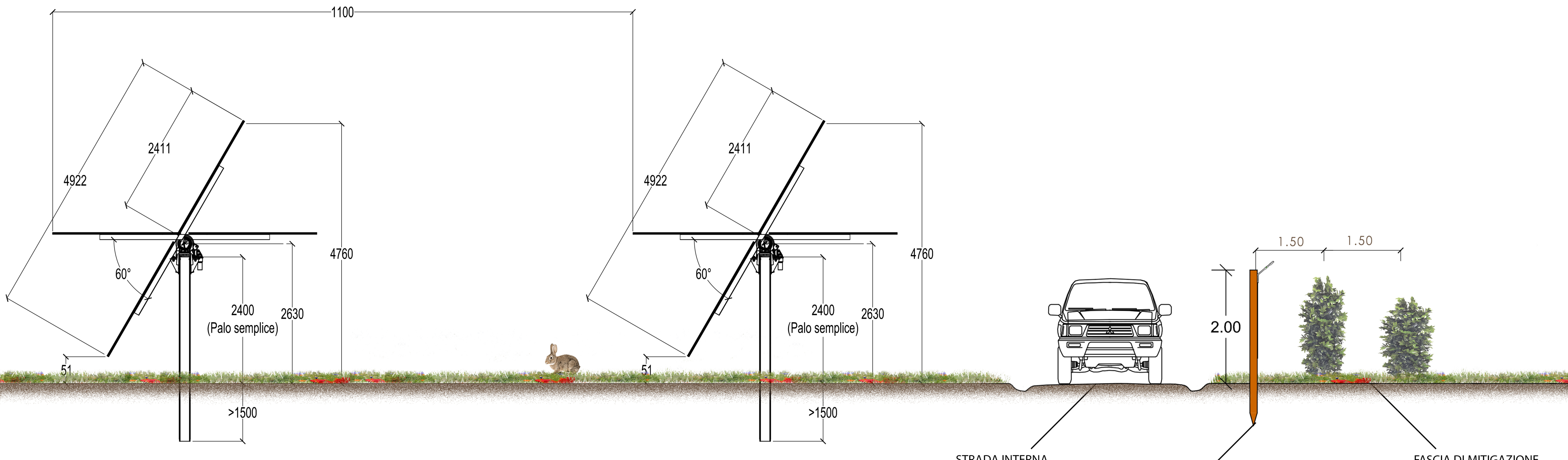
SEZIONE TIPO A-A' Scala 1:50
