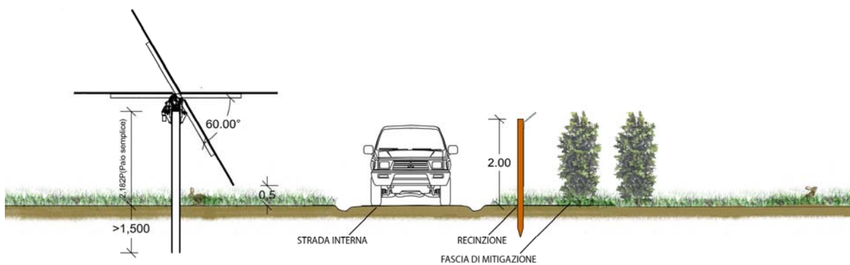
Figura 10 – Fascia di “protezione visiva” – PROSPETTO
