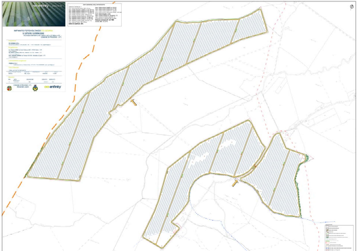
Figura 7 – Impianto EG GEMMA
