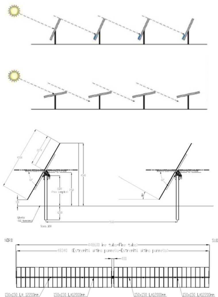
Figura 6 – Moduli su strutture tracker e stringa
