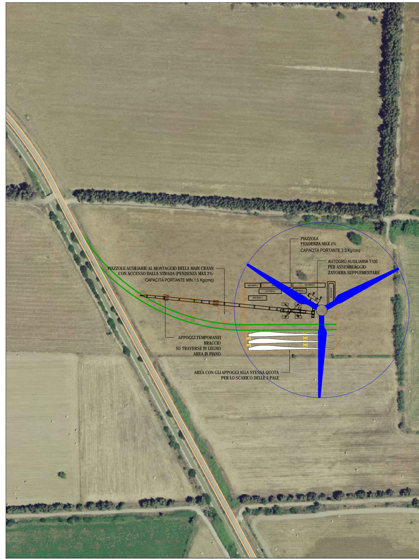
AG01 - PIAZZOLA E VIABILITA' IN FASE DI MONTAGGIO
