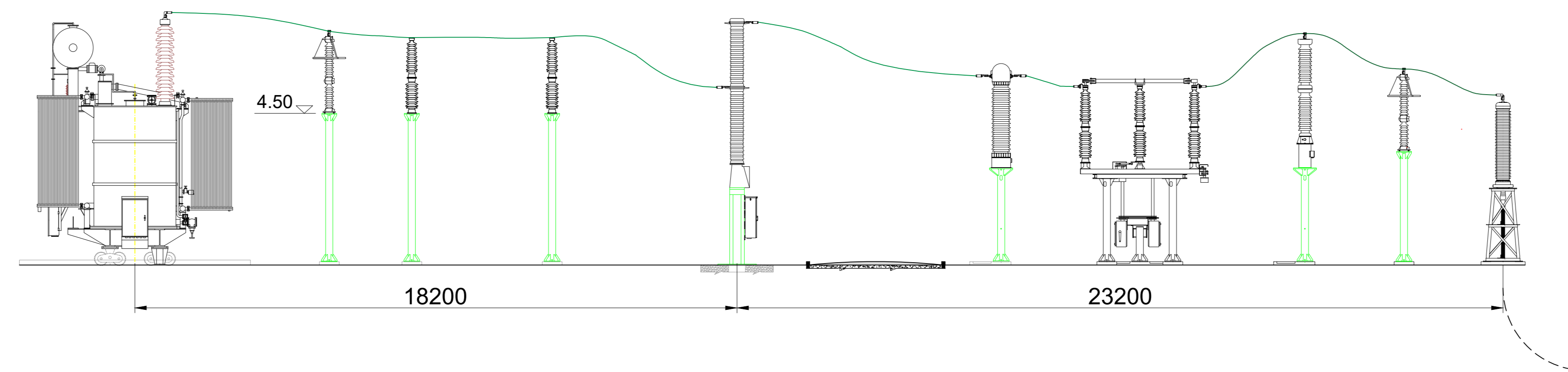
Sezione elettromeccanica stallo arrivo linea e TR 230/36 kV
