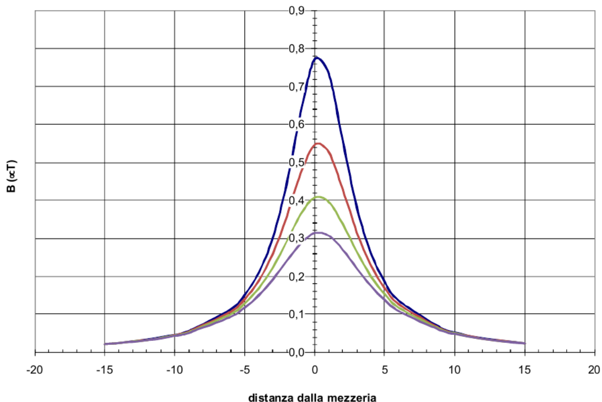
Figura 2. Andamento del campo magnetico in funziona della distanza di interrimento (Blu= 0.5m, rosso=1.0 m, verde=1.5m, viola =2m)
