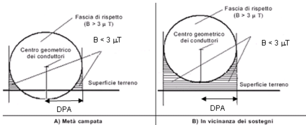
Figura 1 - Schema Fasce di rispetto e DPA in corrispondenza di metà campata e in
