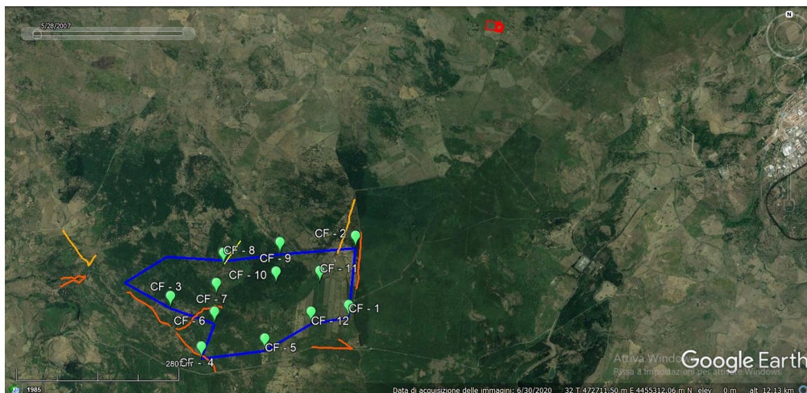
Figura 4. L'Area del Monitoraggio intensivo (Lay-out degli aerogeneratori) ed in alto il punto di realizzazione e collocazione della Sottostazione.
