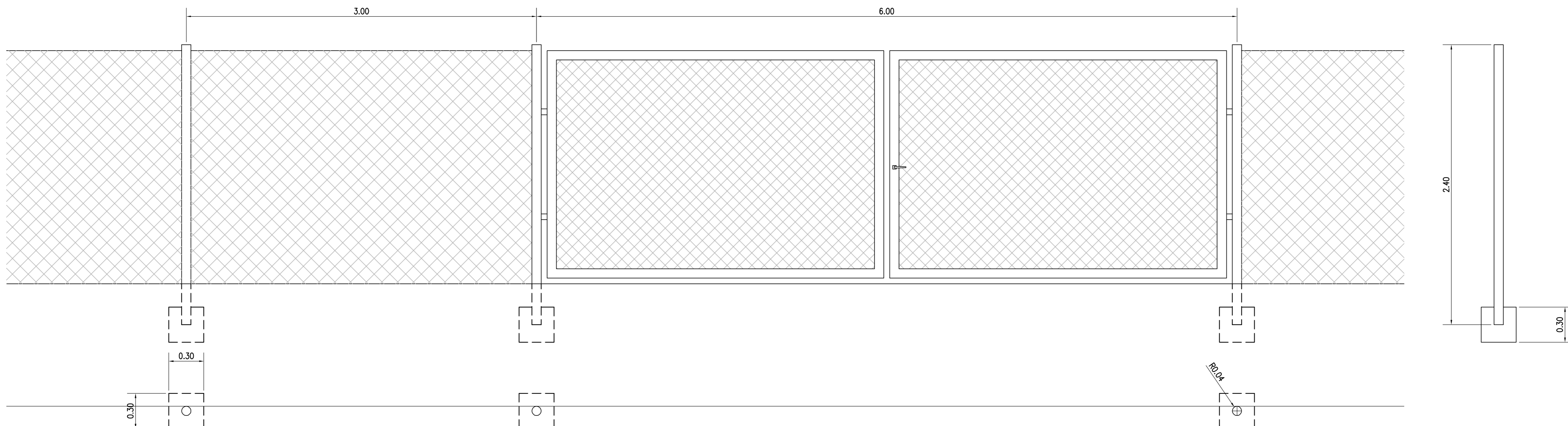
PARTICOLARI RECINZIONE (SCALA 1:20)
