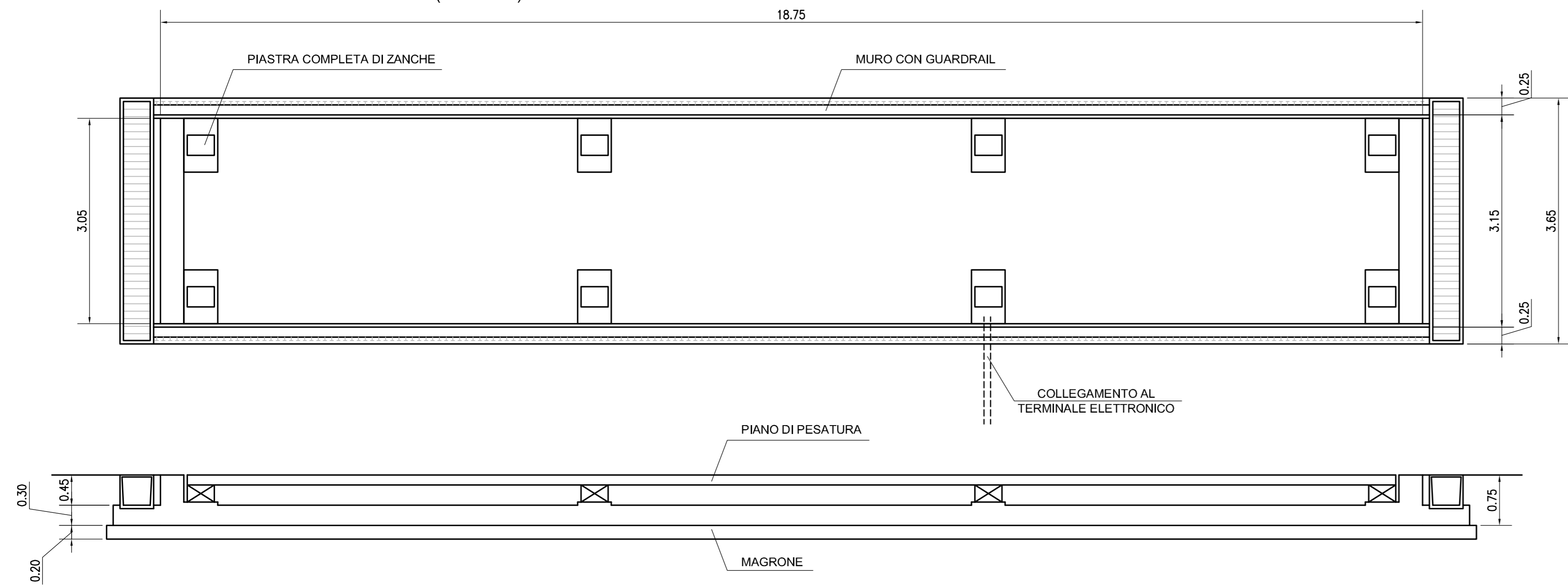
PARTICOLARE DELLA PESA - PIANTE E SEZIONI (scala 1:50)
