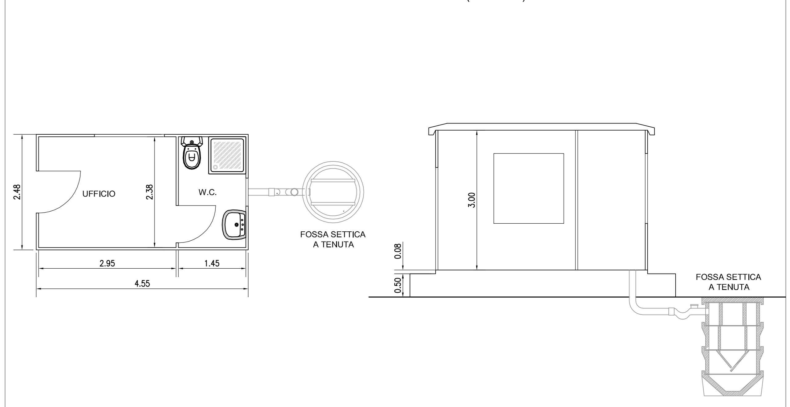
PARTICOLARE DELL'UFFICIO E DELLA FOSSA SETTICA - PIANTE E SEZIONE (scala 1:50)
