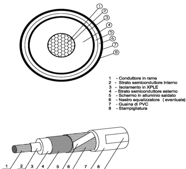
Figura 1. Schema tipo del cavo 150 kV
