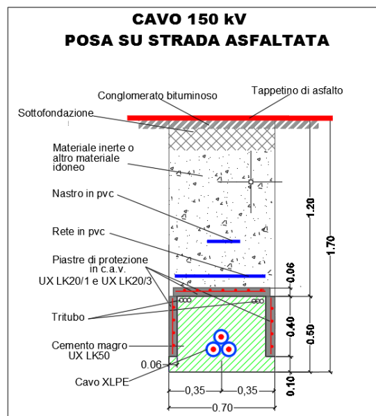
Figura 2: Posa cavo 150 kV
